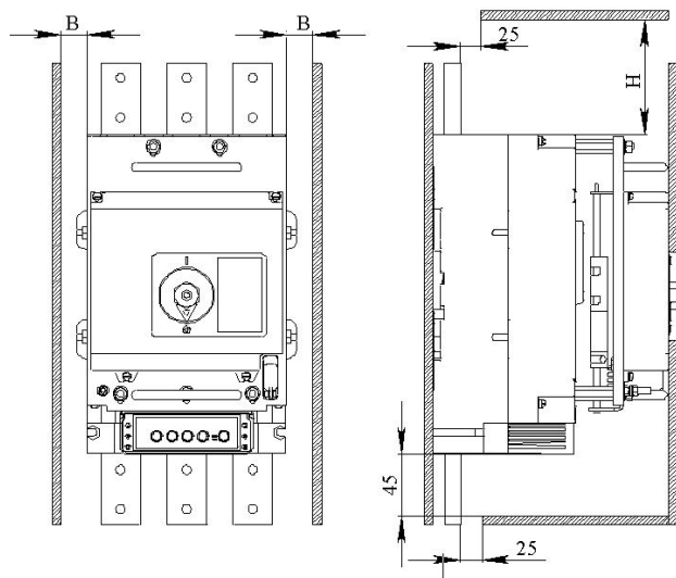
Рисунок Д.2 – Автоматический выключатель с электромагнитным приводом.
