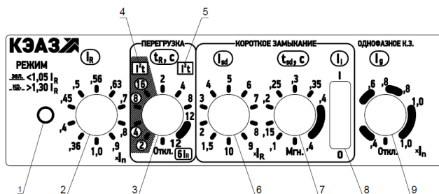
Рисунок 1 – Автоматический выключатель ВА55-41 стационарного исполнения
