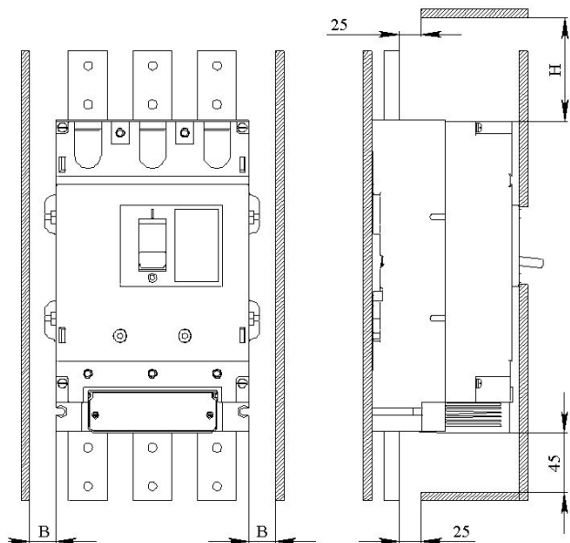
Рисунок Д.1 – Автоматический выключатель с ручным приводом
