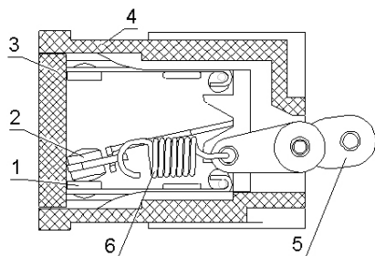
Рисунок 4 – Вспомогательный контакт.
