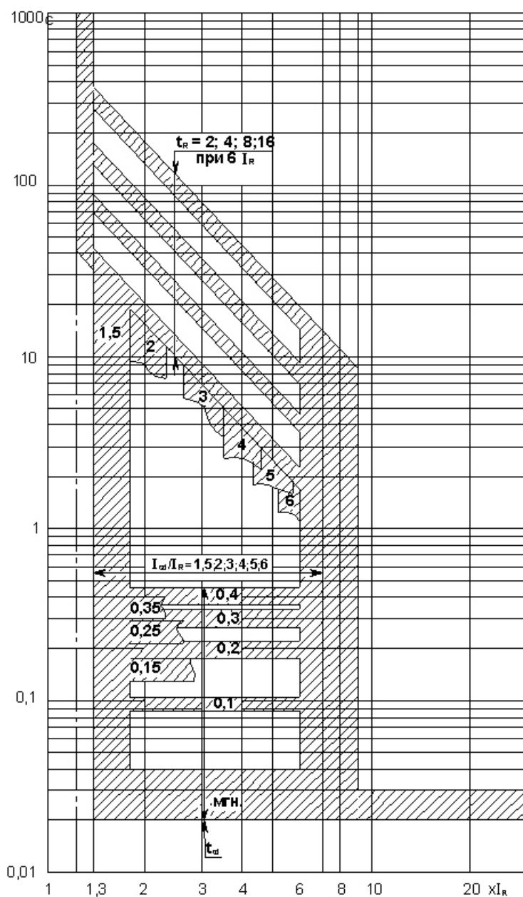
Рисунок В.1 – Выключатель ВА53-41. Обратно-квадратичная зависимость
