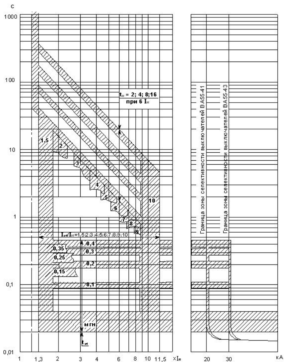
Рисунок В.3 – Выключатель BA55-41. Обратно-квадратичная зависимость
