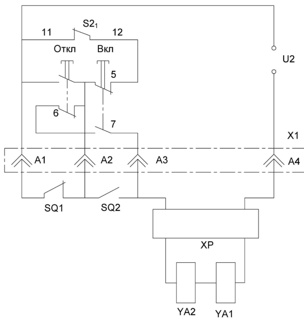
Рисунок Г.5 – Электромагнитный привод постоянного тока
