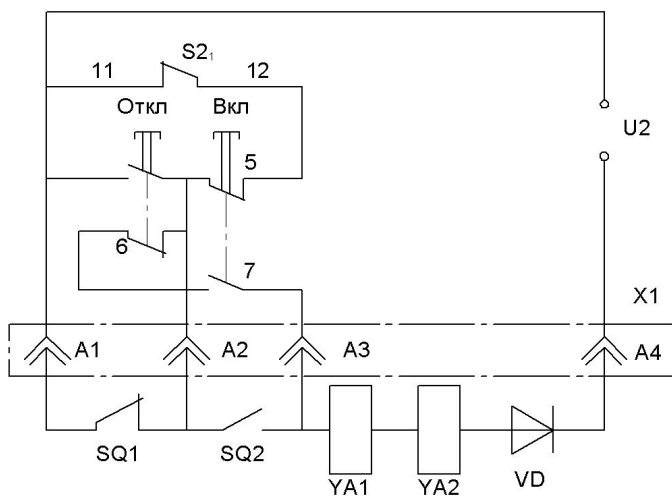
Рисунок Г.4 – Электромагнитный привод переменного тока
