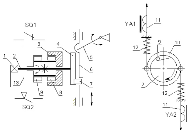
Рисунок 6 – Кинематическая схема электромагнитного привода.
