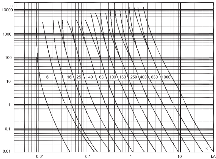
Зона время-токовых характеристик
