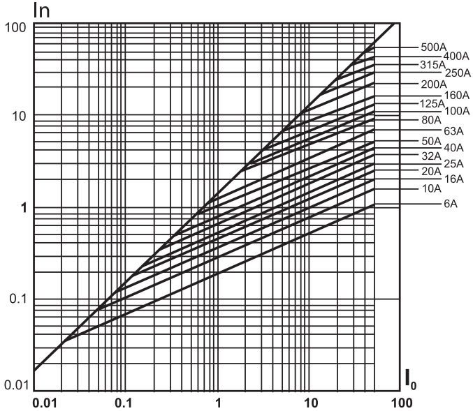
Характеристики пропускаемого тока
