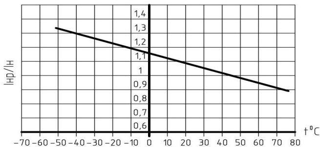
Рисунок А.3 – Зависимость номинального рабочего тока выключателей с приёмкой РС от температуры окружающего воздуха
