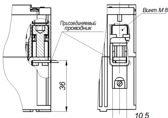
Рисунок 2 – Способы присоединения внешних проводников к выключателю
