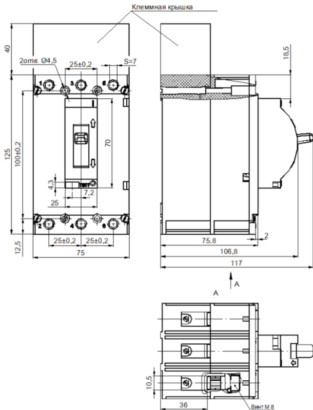
Рисунок Б.1 – Габаритные, установочные, присоединительные размеры и масса выключателя
