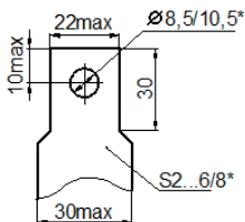
Форма и размеры присоединяемой шины
