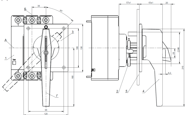
Рисунок Б.2 – Выключатель с ручным дистанционным приводом для оперирования через дверь распределительного устройства
