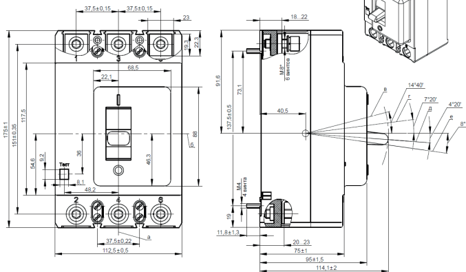
Рисунок Б.1 – Выключатель с ручным приводом: а) выключатель; б) выключатель с клеммной крышкой.
