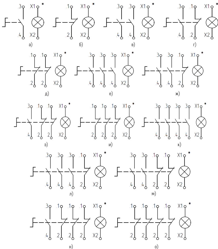
Рисунок Б.3 – Переключатели с самовозвратом
