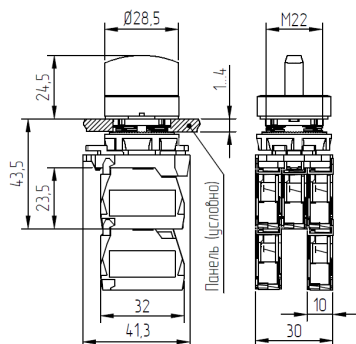
Рисунок А.12 – Переключатели КПЕ16...Р, КПЕ21...Р, КПЕ26...Р
