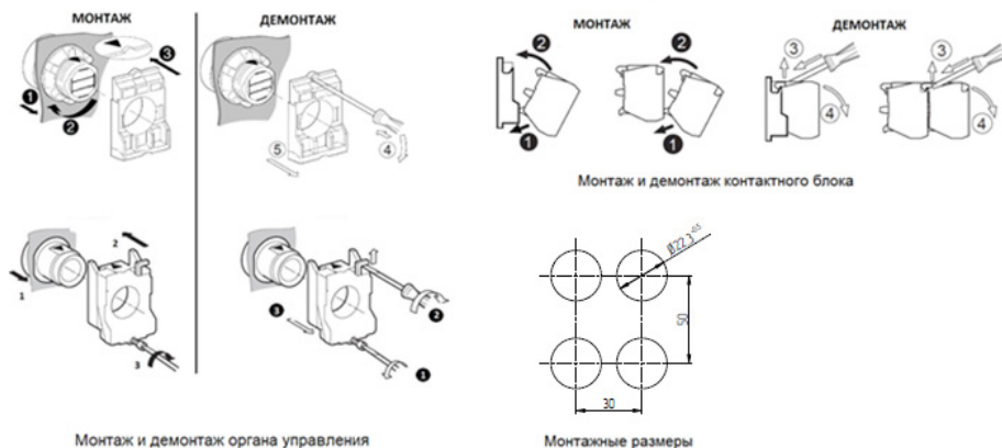
Рисунок 1 – Схема монтажа и демонтажа выключателей
