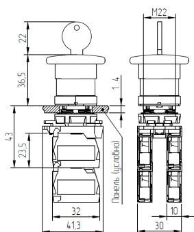
Рисунок А.5 – Выключатели КМЕ51...мФ, КМЕ55...мФ, КМЕ56...мФ
