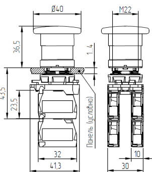
Рисунок А.5 – Выключатели КМЕ51...мФ, КМЕ55...мФ, КМЕ56...мФ
