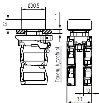
Рисунок А.9 – Выключатели КМЕ45...МЛС, КМЕ46...МЛС
