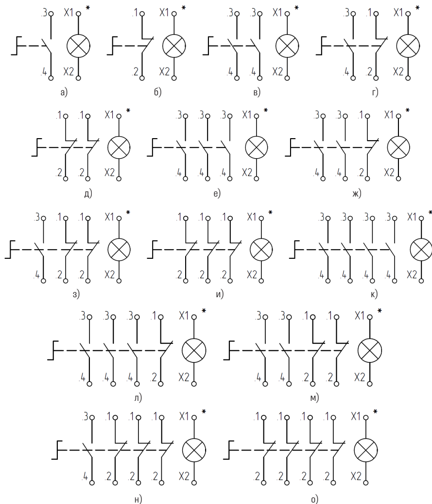
Рисунок Б.1 – Выключатели с самовозвратом
