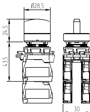
Рисунок А.12 – Переключатели КПЕ16...Р, КПЕ21...Р, КПЕ26...Р
