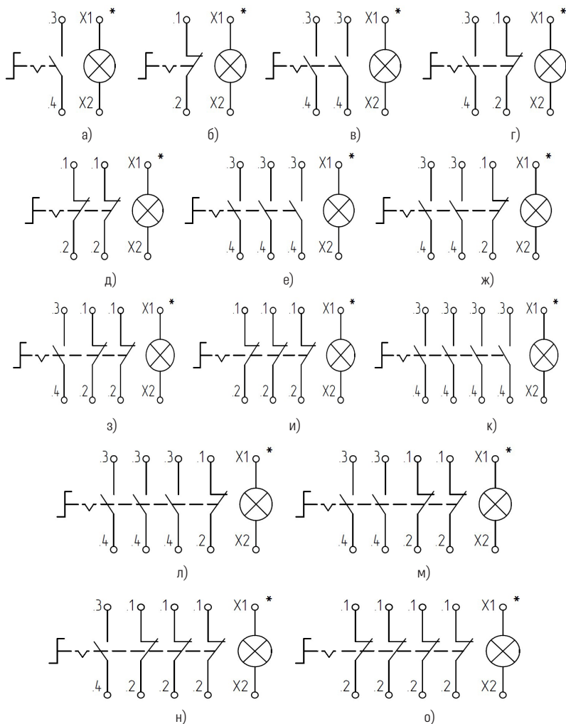
Рисунок Б.4 – Переключатели с фиксацией
