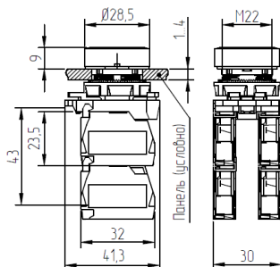
Рисунок А.1 – Выключатели КМЕ41...м, КМЕ45...м, КМЕ46...м
