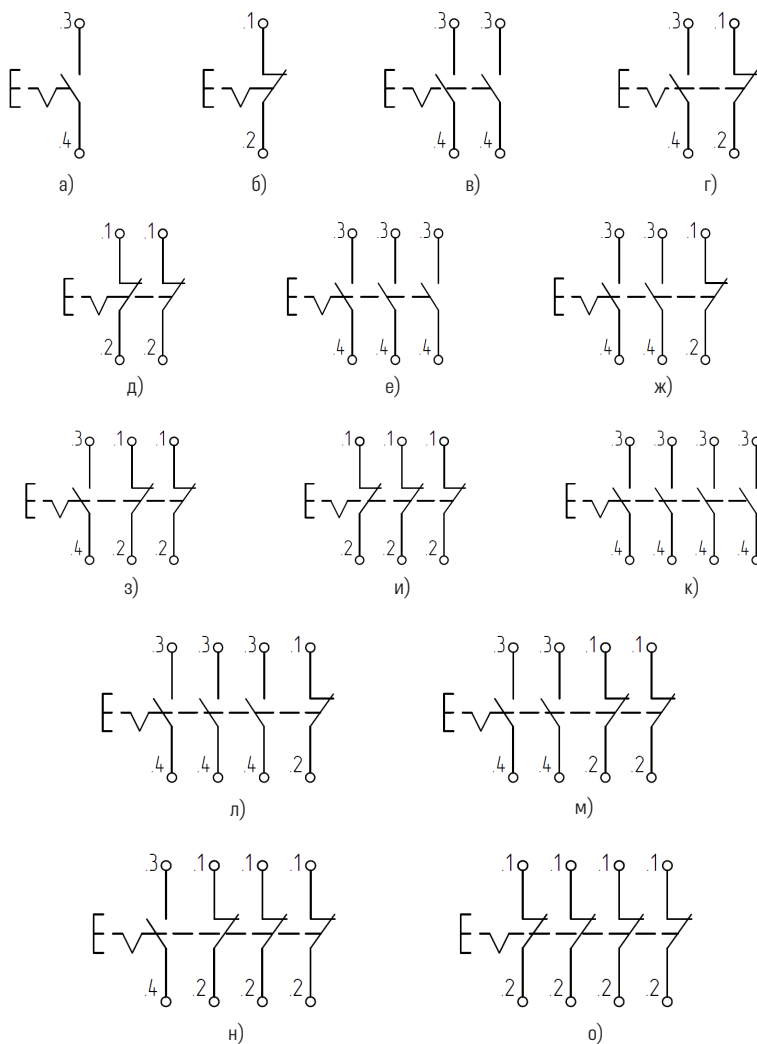
Рисунок Б.2 – Выключатели аварийного останова
