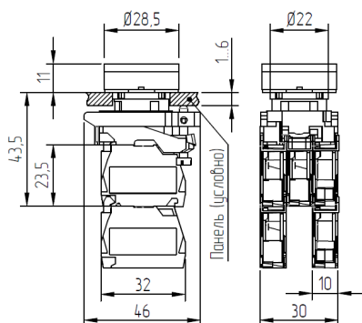
Рисунок А.9 – Выключатели КМЕ45...МЛС, КМЕ46...МЛС
