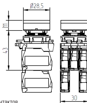
Рисунок А.2 – Выключатели КМЕ41...мЛ, КМЕ45...мЛ, КМЕ46...мЛ
