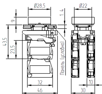
Рисунок А.7 – Выключатели КМЕ41...МС, КМЕ45...МС, КМЕ46...МС
