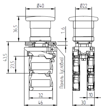
Рисунок А.10 – Выключатели КМЕБ1...мФС, КМЕБ5...мФС, КМЕБ6...мФС
