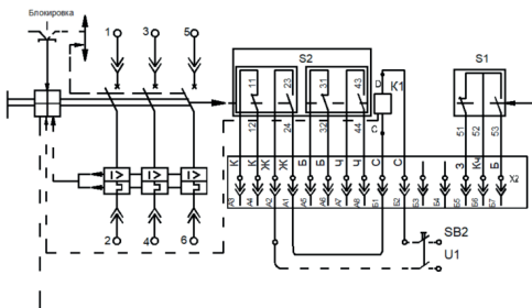
Рисунок Г.7 – Схема электрическая принципиальная выключателей выдвжного исполнения, с нулевым или минимальным расцепителем напряжения, вспомогательными контактами сигнализации автоматического отключения, вспомогательными контактами и электромагнитным приводом
