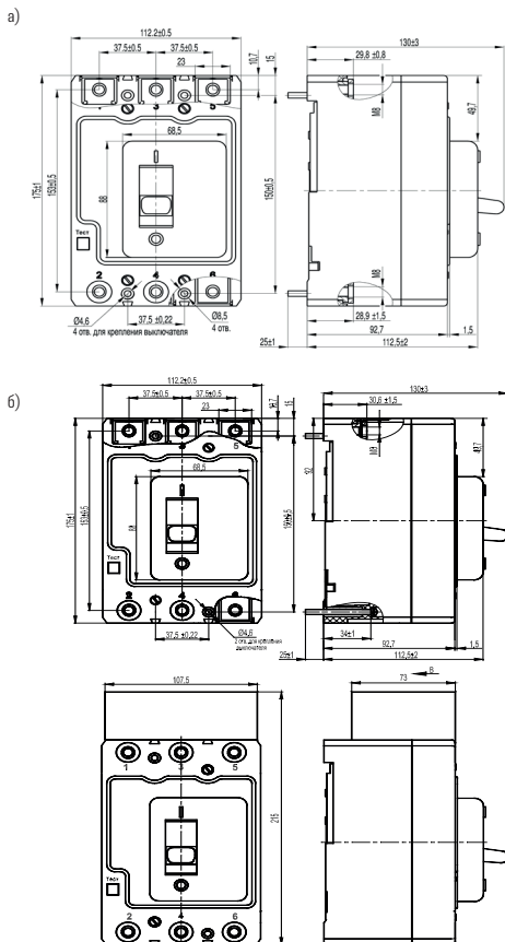
Рисунок Б.1 – Выключатель с зажимами для переднего присоединения
