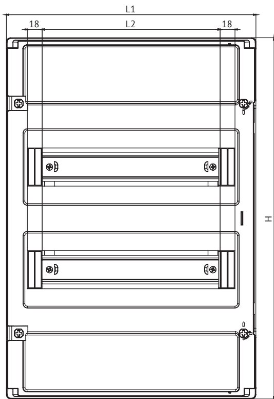
Вид спереди
