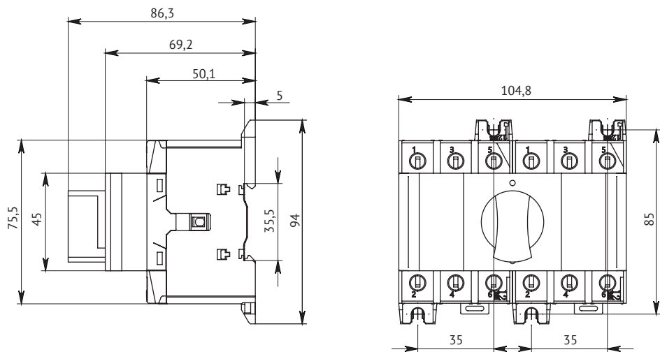
Рисунок А.7 – OptiSwitch DI-DC реверсивный разъединитель на номинальный ток от 16 до 100 А
