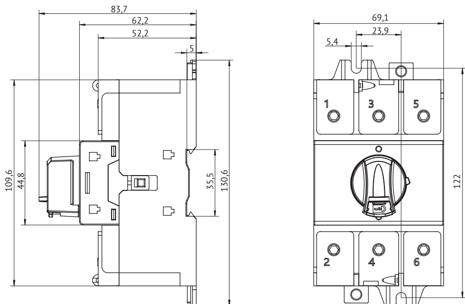
Рисунок А.5 – OptiSwitch DI-DC на номинальный ток 125 А в трехполюсном исполнении
