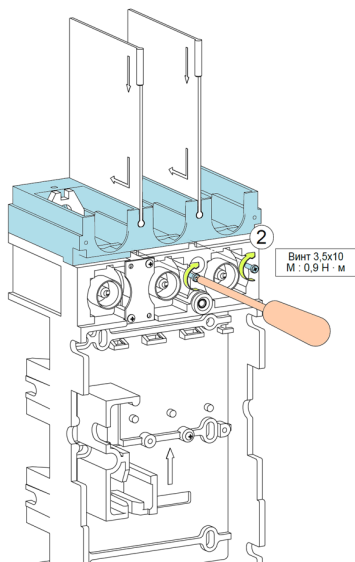
б) OptiMat D400, D630
