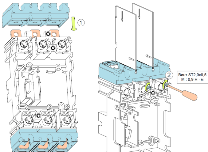
а) OptiMat D100, D160, D250
