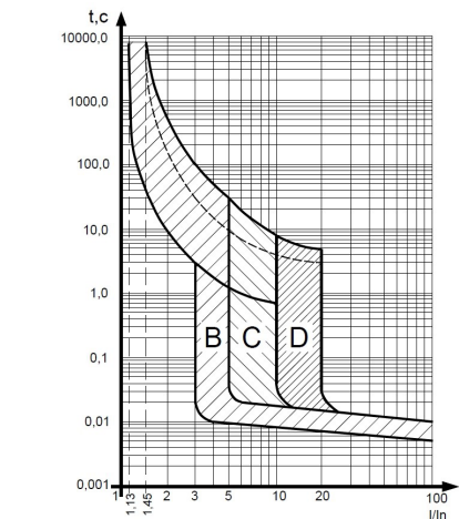
Рисунок Б.1 Пунктирная линия – верхняя граница время-токовой характеристики для автоматических выключателей с номинальным током I_n \leq 32A .
