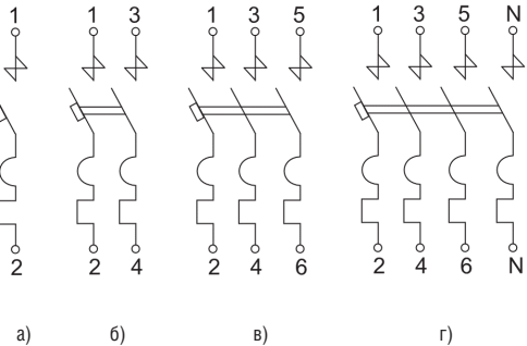
а) однополюсного; б) двухполюсного с двумя защищенными полюсами; в) трехполюсного с тремя защищенными полюсами; г) четырехполюсного с четырьмя защищенными полюсами.
