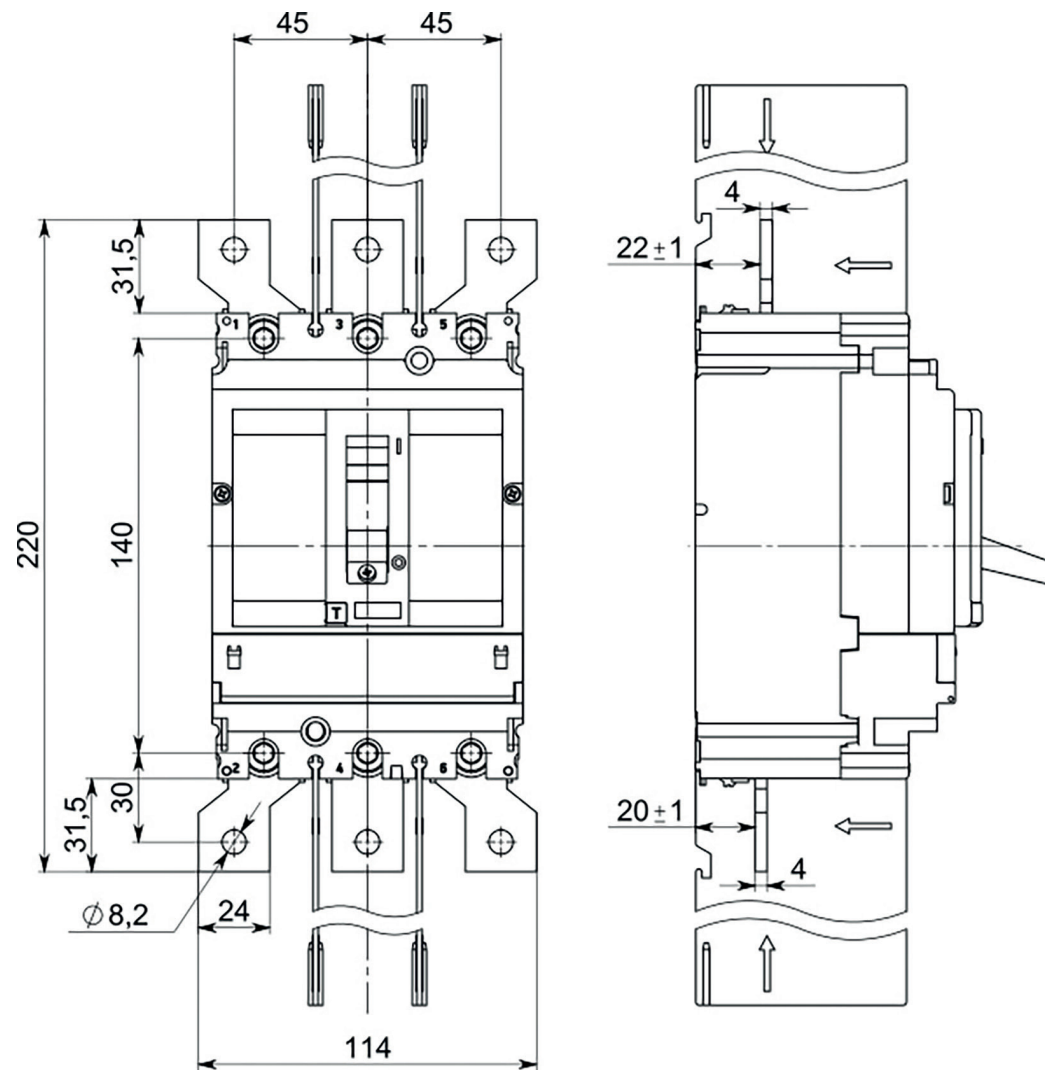
Рисунок 2 – Габаритные, установочные и присоединительные размеры выключателей OptiMat D100, D160, D250 с расширителями полюсов
