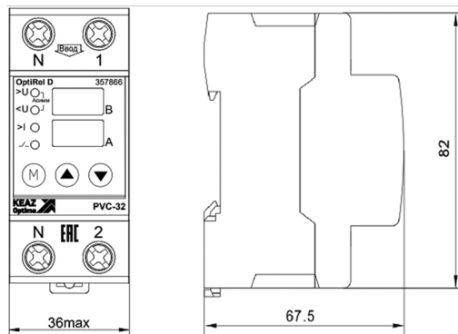
Рисунок А.1 – Габаритные размеры реле
