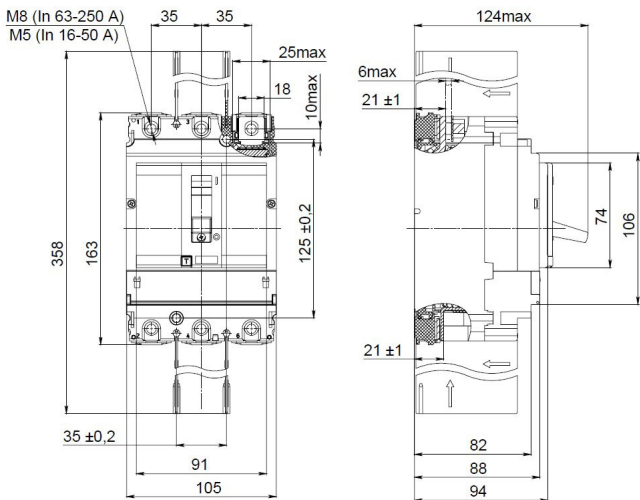
Рисунок 8 – Габаритные, установочные и присоединительные размеры выключателя
