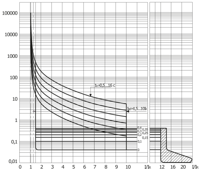
Рисунок 2 – Время-токовая характеристика выключателей с микропроцессорным расцепителем
