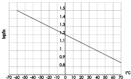
Рисунок 4 – Зависимость номинальных рабочих токов выключателей с термомангнитными регулируемыми расцепителями от температуры окружающей среды
