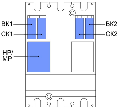
Рисунок 10 – Схема расположения гнезд под вспомогательные
