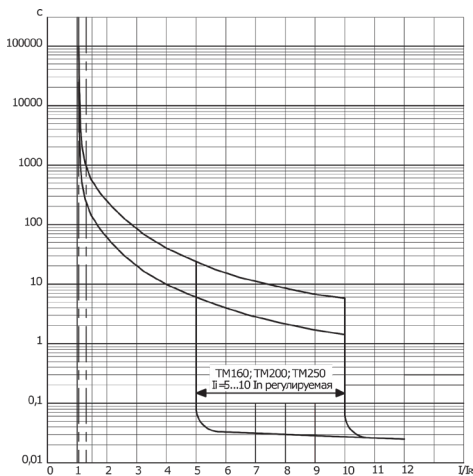
Рисунок 7 – Время-токовые характеристики выключателей OptiMat D250-TM160; OptiMat D250-TM200; OptiMat D250-TM250 с регулируемой уставкой по току расцепителей токов короткого замыкания
