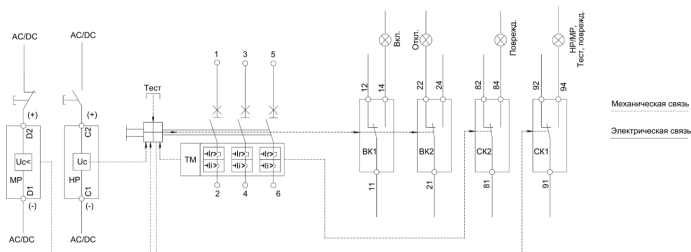
б) с термагнитными регулируемые расцепителями
