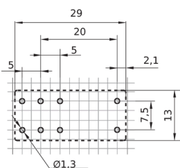
Рисунок Б.3 – Установочные размеры для печатного монтажа для реле OptiRel G RP40-52 и OptiRel G RP40-61 с CO контактами
