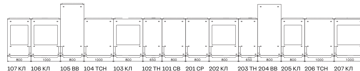
Фронтальный вид и вид сверху ЗРУ-6 кВ
