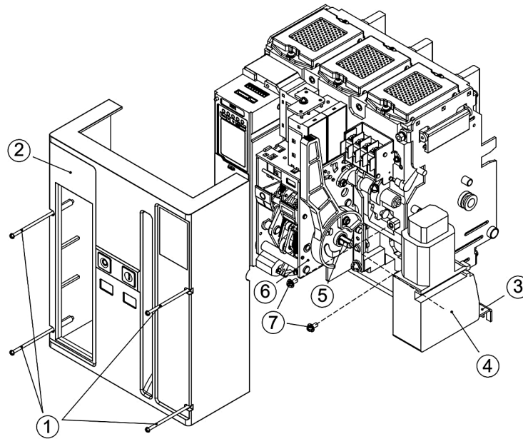
1-Винты, 2-Лицевая панель, 3-Монтажная пластина, 4-Мотор-редуктор, 5-Кулачковый вал, 6-Механизм свободного расцепления, 7-Винты M4x10
