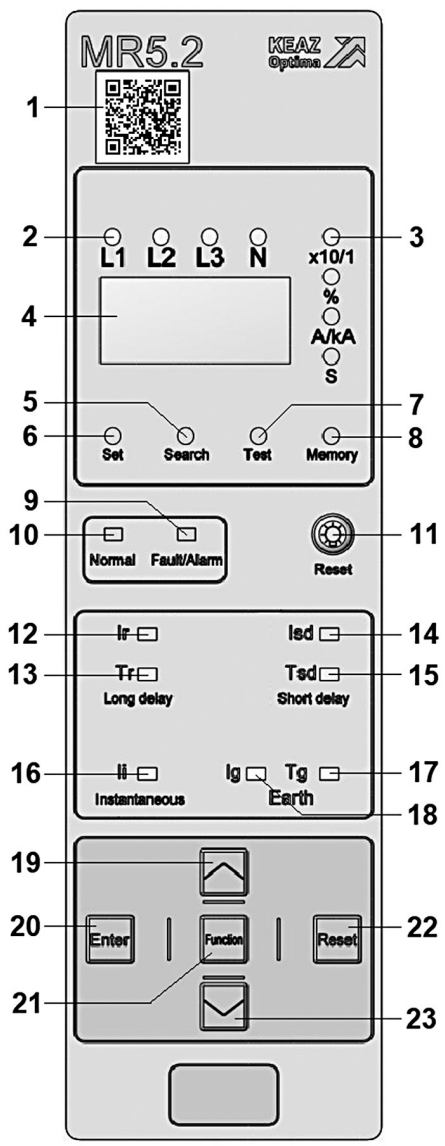
Рисунок 3 – Микропроцессорный расцепитель MR5.2
