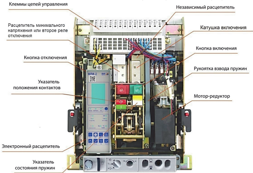
Рисунок 1 – Выключатель выдвижного исполнения OptiMat A-S1
