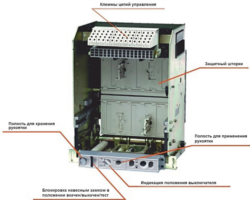
Рисунок 2 – Корзина выдвижного выключателя OptiMat A-S1
