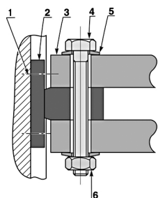
Рисунок В.5 – Присоединение шин к выключателю
