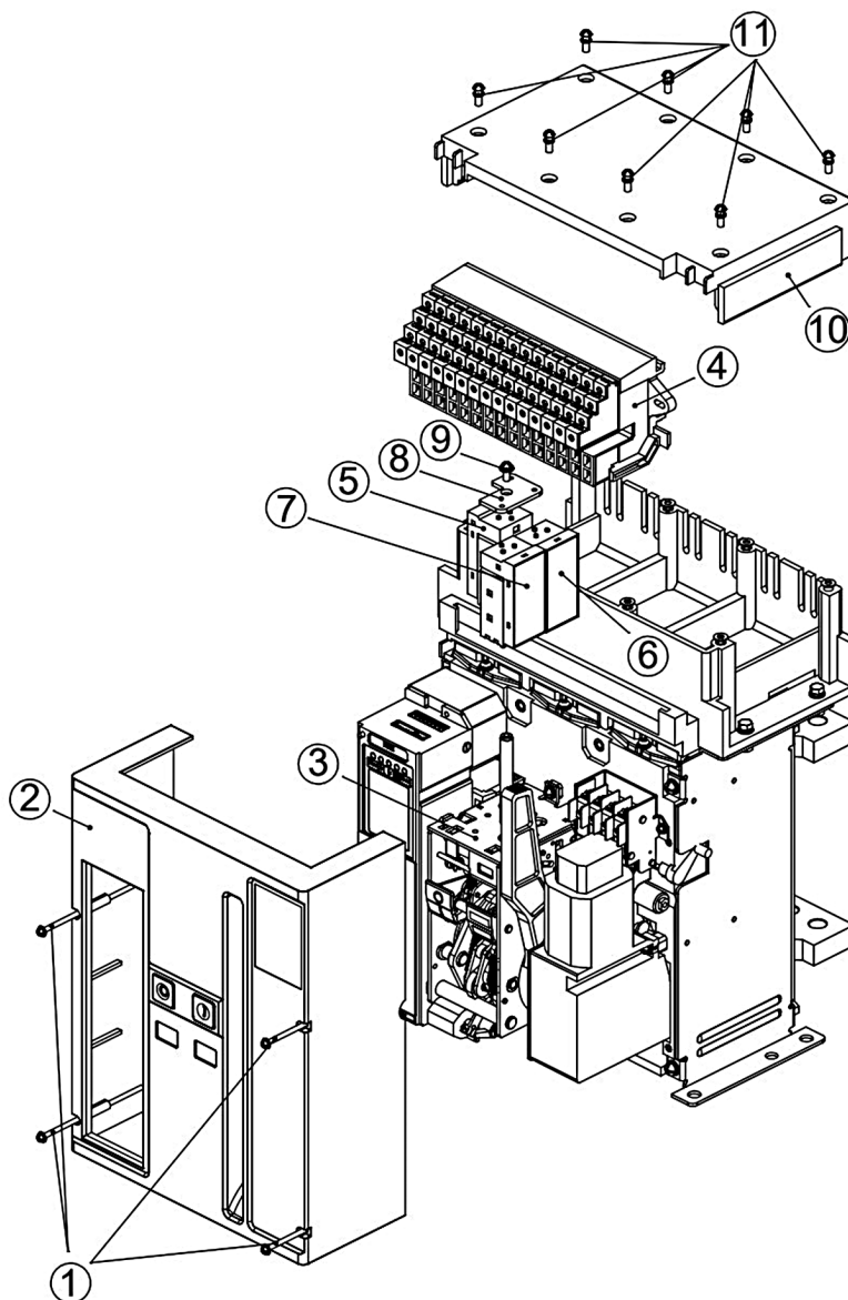
1-Винты, 2-Лицевая панель, 3-Механизм свободного расцепления, 4- Клеммная колодка, 5- Расцепитель минимального напряжения или второй независимый расцепитель, 6- Независимый расцепитель, 7- Катушка включения, 8-Пластина, 9-Винт, 10-Крышка, 11-Винты
