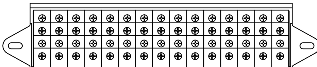
Рисунок Б.3 - Клеммы цепей управления стационарного и выдвижного выключателя OptiMat A-S1 с указанием нумерации.
