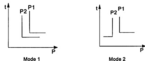
Рисунок 15 – Режим контроля нагрузки по мощности
