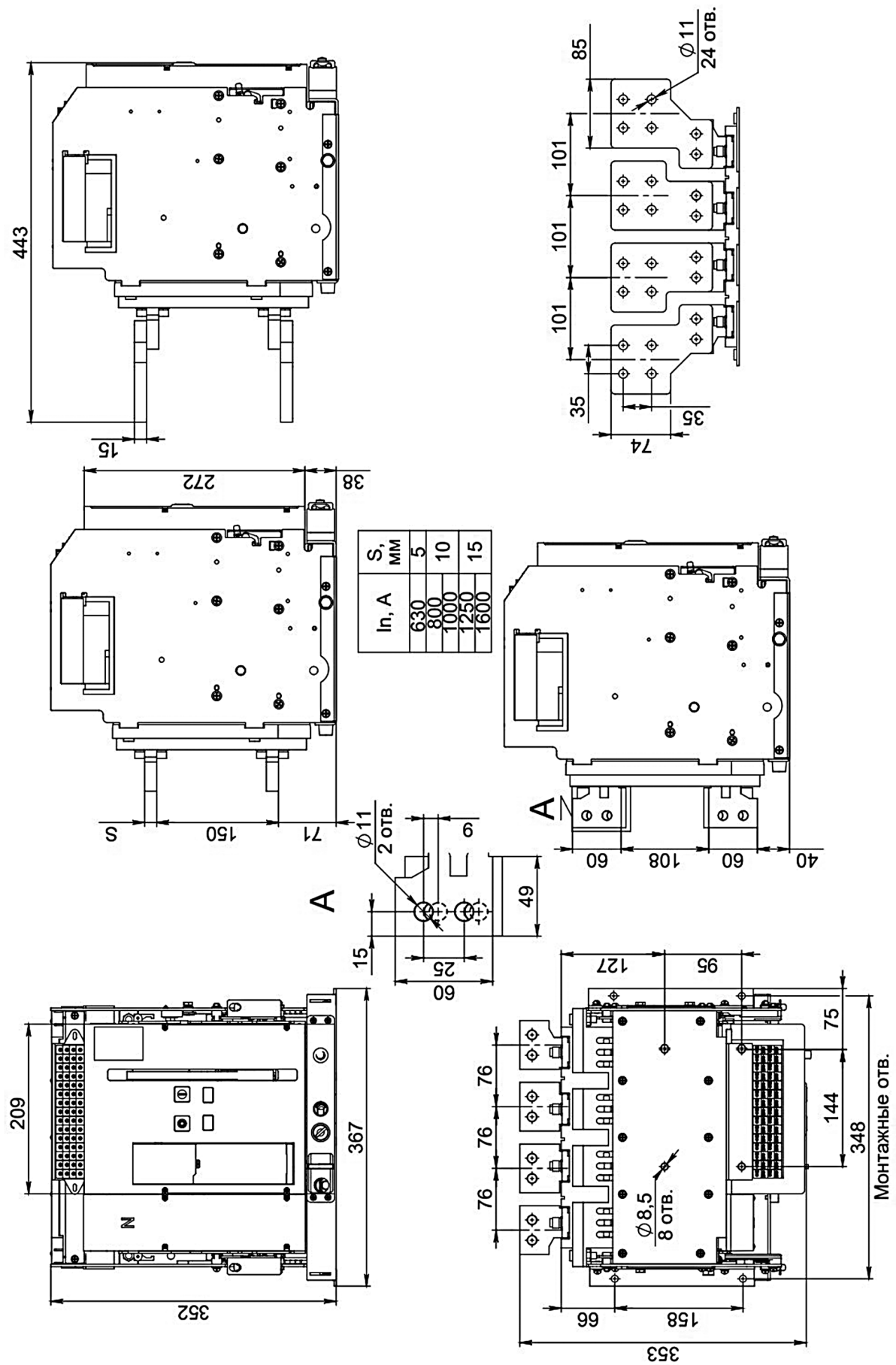
Рисунок А.2 - Габаритные размеры четырехполюсных выключателей OptiMat A выдвигного исполнения на токи до 1600 А
