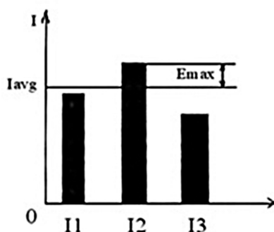
Рисунок 10 – Перекос фаз
