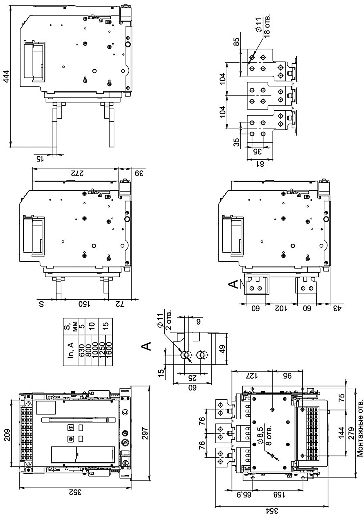
Рисунок А.1 - Габаритные размеры трехполюсных выключателей OptiMat A выдвигного исполнения на токи до 1600 А
