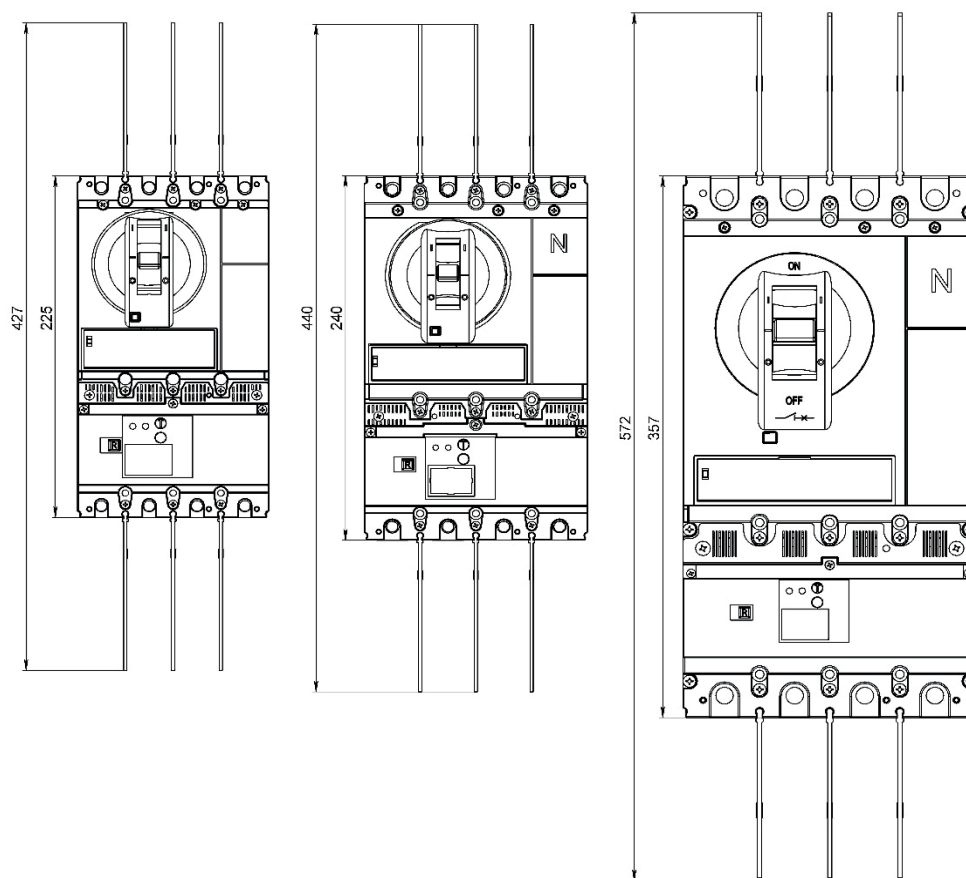
Рисунок 21 – Габаритные размеры выключателей OptiMat T125, T250, T400 (T630) с блоком защиты от токов утечки.
