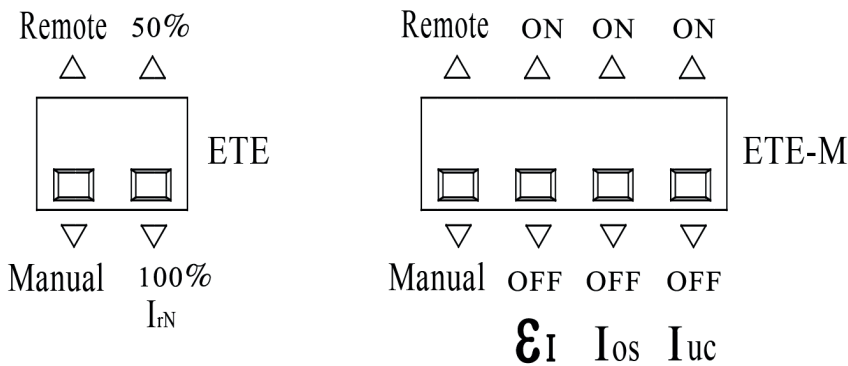
Рисунок 7 – DIP-переключатели режимов настройки уставок и режима защиты нейтрали (для расцепителя ETE), режимов настройки уставок, активации защит от небаланса тока, затянутого пуска и минимального тока (для расцепителя ETE-M)
