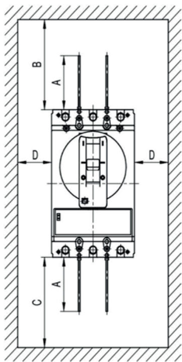
Рисунок 22 – Изоляционные расстояния для выключателей OptiMat T с передними выводами и межфазными перегородками
