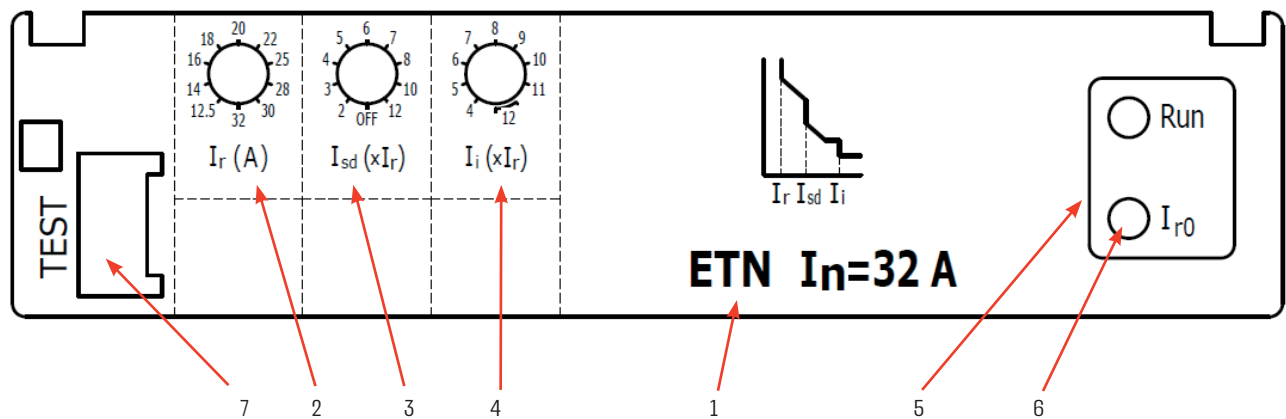
Рисунок 1 – Пример лицевой панели расцепителя защиты ETN
