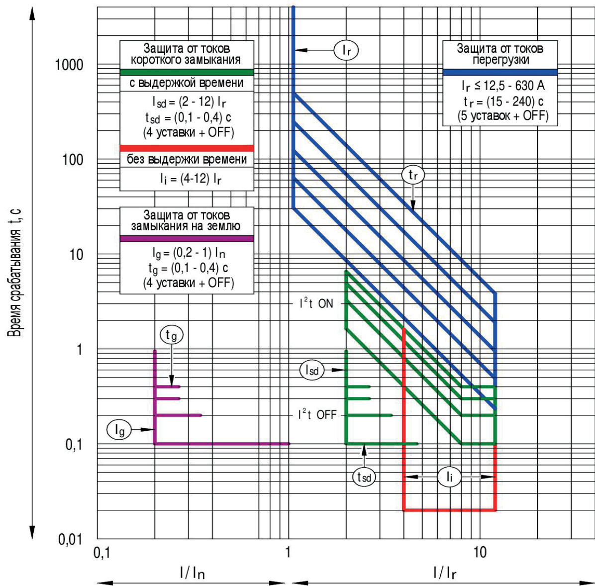
Рисунок Б.3 — Время-токовые характеристики выключателей с электронными регулируемыми расцепителями типов ETA, ETA-COM, ETE для защиты распределительных сетей
