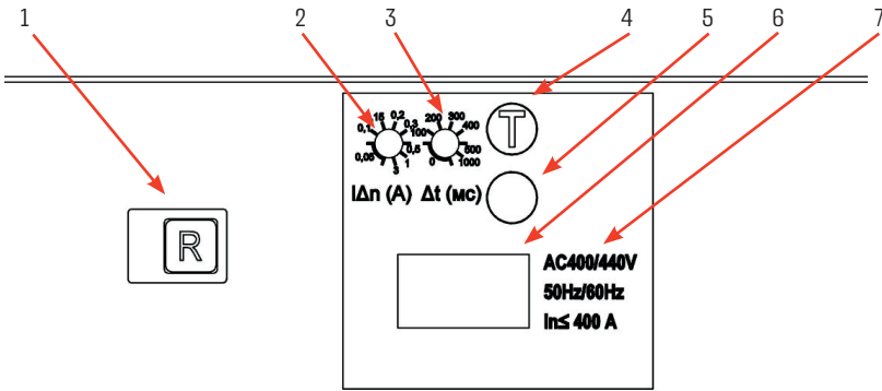
Рисунок 17 – Лицевая панель блока защиты от токов утечки RC.
