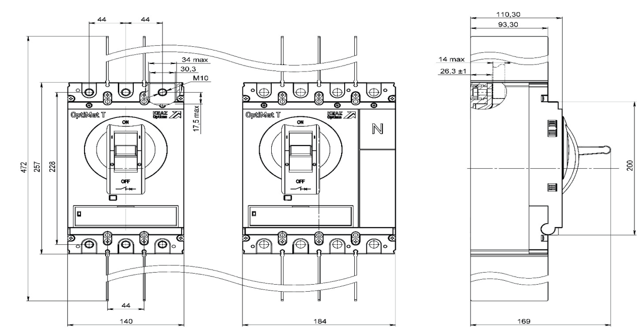
Рисунок 20 – Габаритные размеры выключателей OptiMat T400 (T630) переднего присоединения.
