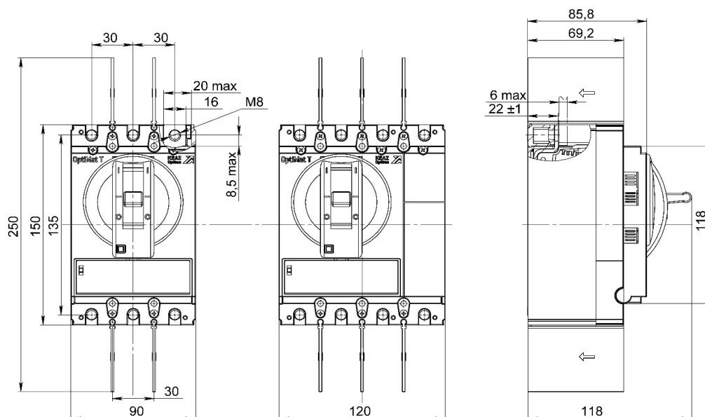
Рисунок 18 – Габаритные размеры выключателей OptiMat T125 (T160) переднего присоединения.
