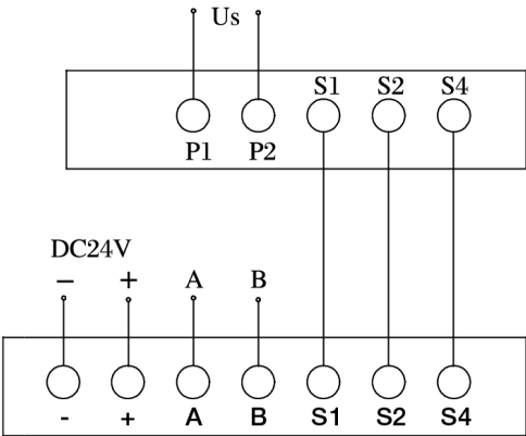
Рисунок 16 – Схема подключения специального кабеля связи и управления ESMO-COM и моторного привода ESMO
