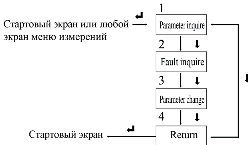
Рисунок 10 – Основное меню расцепителя ETE
