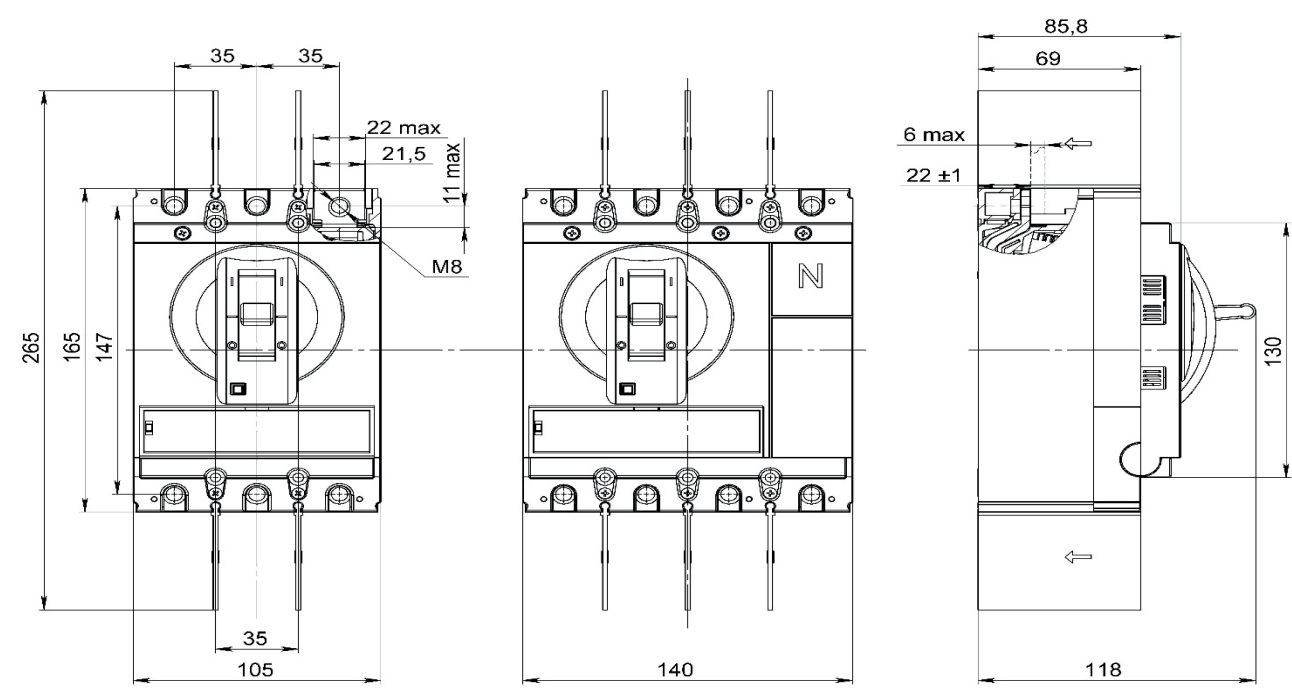
Рисунок 19 – Габаритные размеры выключателей OptiMat T250 переднего присоединения.
