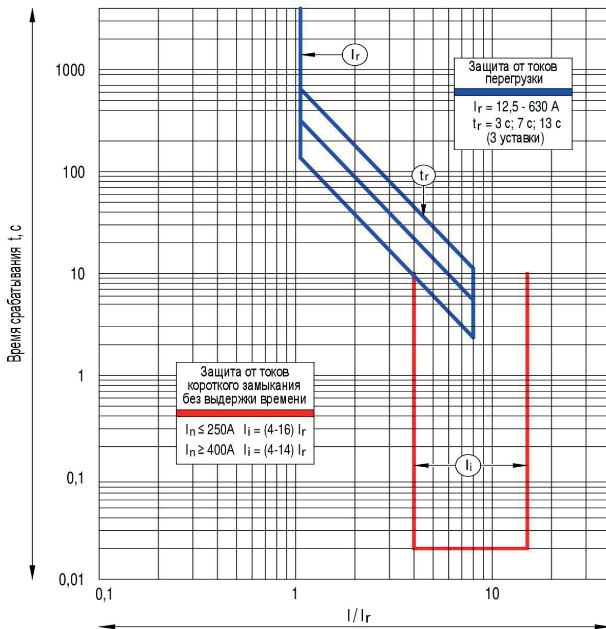
Рисунок Б.2 — Время-токовые характеристики выключателей с электронными регулируемым расцепителями типа ETN-M для защиты электродвигателей
