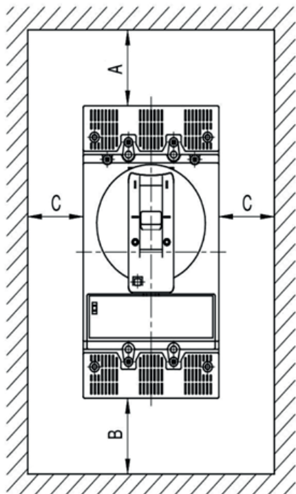
Рисунок 23 – Изоляционные расстояния для выключателей OptiMat T с задними выводами и крышками выводов
