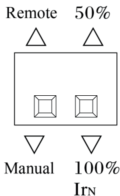
Рисунок 3 – DIP-переключатели режимов настройки уставок и режима защиты нейтрали
