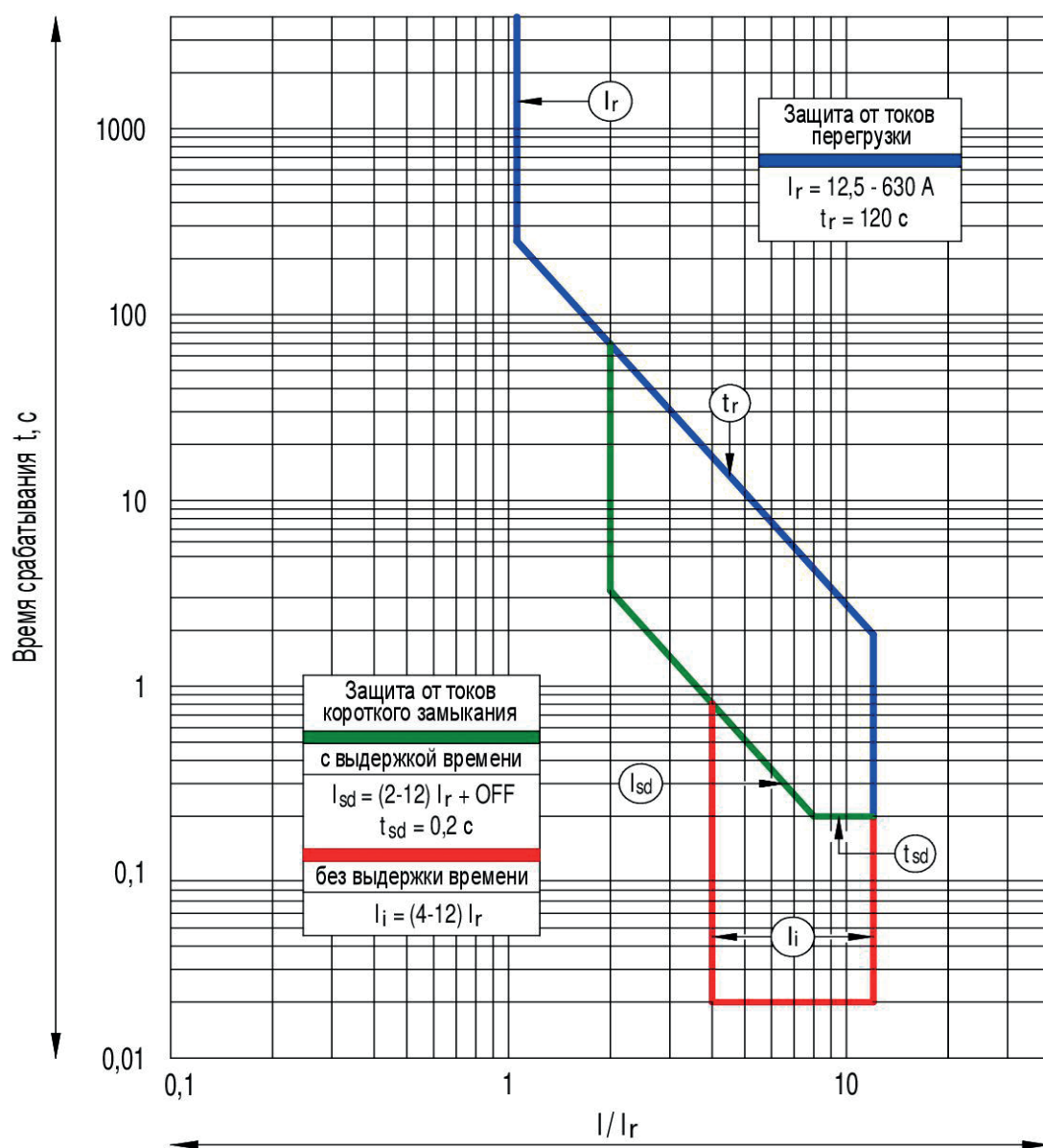
Рисунок Б.1 — Время-токовые характеристики выключателей с электронными регулируемым расцепителями типа ETN для защиты распределительных сетей
