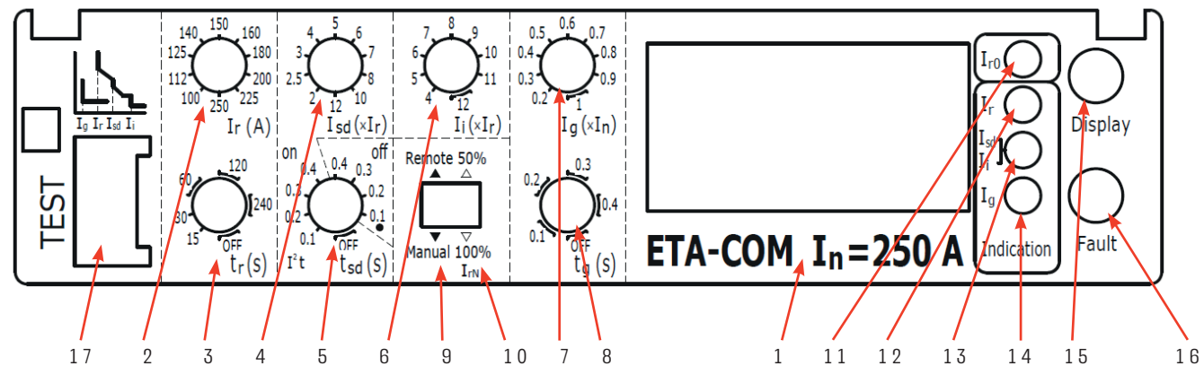
Рисунок 2 – Пример лицевой панели электронного расцепителя ETA-COM
