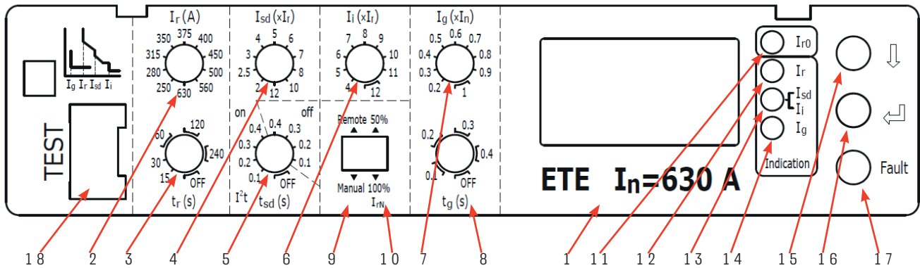
Рисунок 6 – Пример лицевой панели электронного расцепителя ЕТЕ
