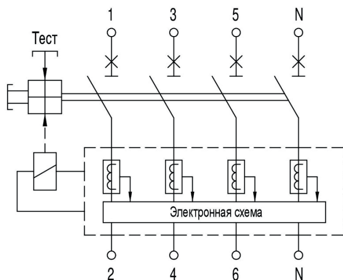
Рисунок Г.2 – Электрическая функциональная схема выключателей с блоком защиты от токов утечки и электронными расцепителями защиты
