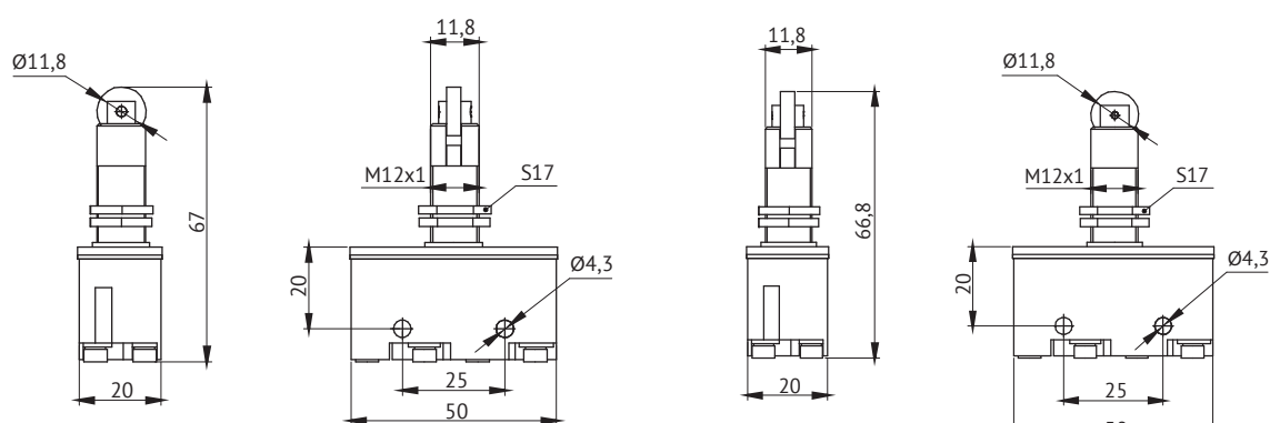
Масса - 0,06 кг Микропереключатель с толкателем с поперечным роликом и степенью защиты IP00
