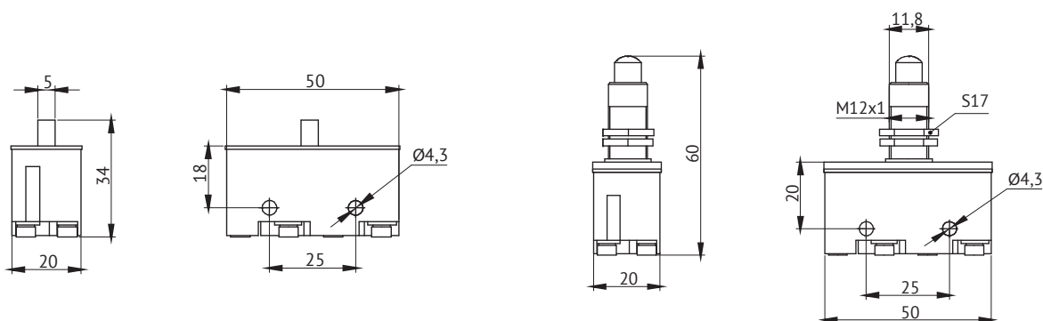
Масса - 0,02 кг Микропереключатель с толкателем и степенью защиты IP00
