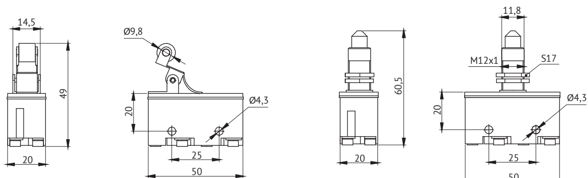
Масса - 0,04 кг Микропереключатель с толкателем с рычагом и роликом и степенью защиты IP00
