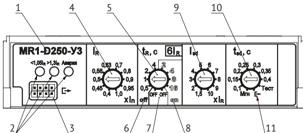
Рисунок 1 - Общий вид лицевой панели микропроцессорного максимального расцепителя тока
