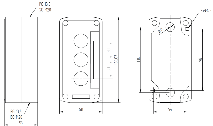
Масса – 0,238 кг Рисунок А.4 – Посты OptiSignal D22 A5-BD-3
