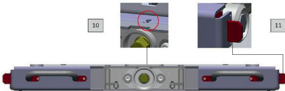
Рисунок 7 – Места смазки подвижных узлов тележки (для выкатного исполнения, обозначения согласно таблице 10)
