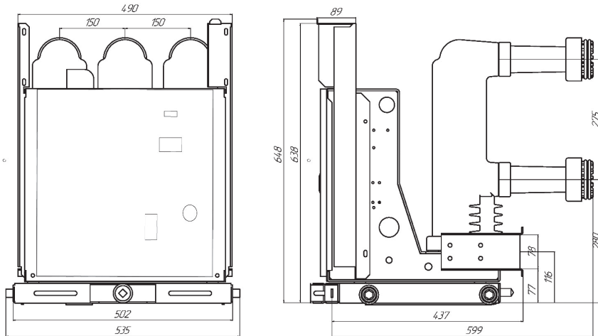
Рисунок В.1 – Габаритные, присоединительные и установочные размеры выключателя типа (передняя панель не изображена) OptiMat ВВ-MD-10-20 (25; 31,5; 40)/630 (1000; 1250)-2-МВ (ММ)-150
