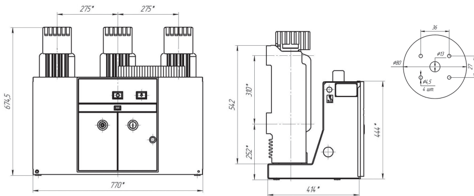
Рисунок А.4 – Габаритные, присоединительные и установочные размеры, масса выключателя типа ВВ-MD-10-31,5 (40; 50)/2000-2-FX-275
