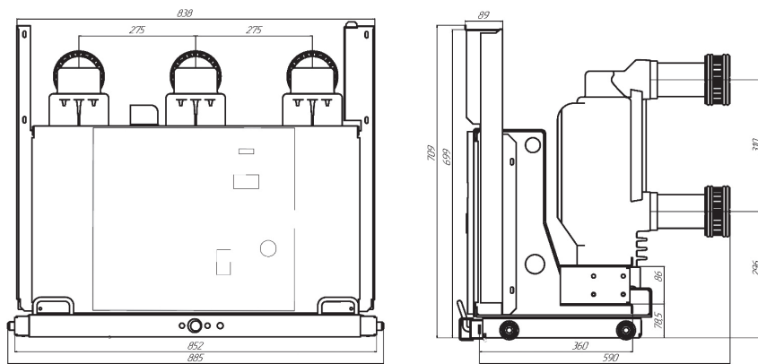
Рисунок В.4 – Габаритные, присоединительные и установочные размеры выключателя типа (передняя панель не изображена) OptiMat BB-MD-10-31,5 (40; 50)/2000-2-MB (MM)-275
