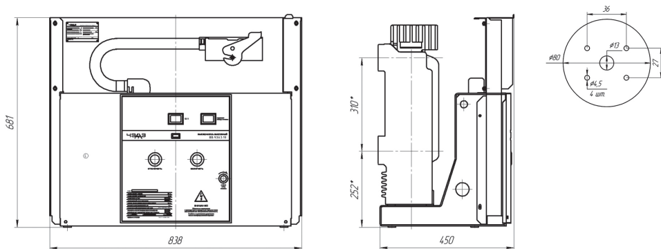
Рисунок А.5 – Габаритные, присоединительные и установочные размеры, масса выключателя типа OptiMat ВВ-MD-10-31,5 (40; 50)/2500 (3150; 4000)-2-FX-275
