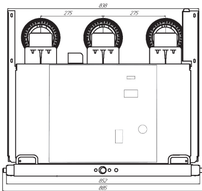
Рисунок В.5 – Габаритные, присоединительные и установочные размеры выключателя типа (передняя панель и радиаторы не изображены) OptiMat BB-MD-10-31,5 (40; 50)/ 2500 (3150; 4000)-2-MB (MM)-275
