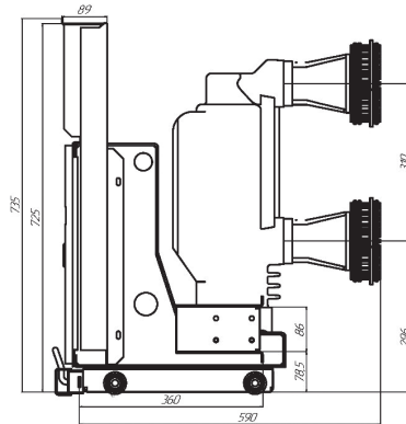
Рисунок В.5 – Габаритные, присоединительные и установочные размеры выключателя типа (передняя панель и радиаторы не изображены) OptiMat BB-MD-10-31,5 (40; 50)/ 2500 (3150; 4000)-2-MB (MM)-275
