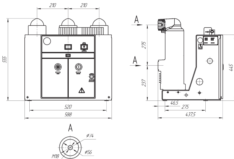
Рисунок А.3 – Габаритные, присоединительные и установочные размеры, масса выключателя типа OptiMat-ВВ-MD-10-20 (25; 31,5; 40)/2000-2-FX-210
