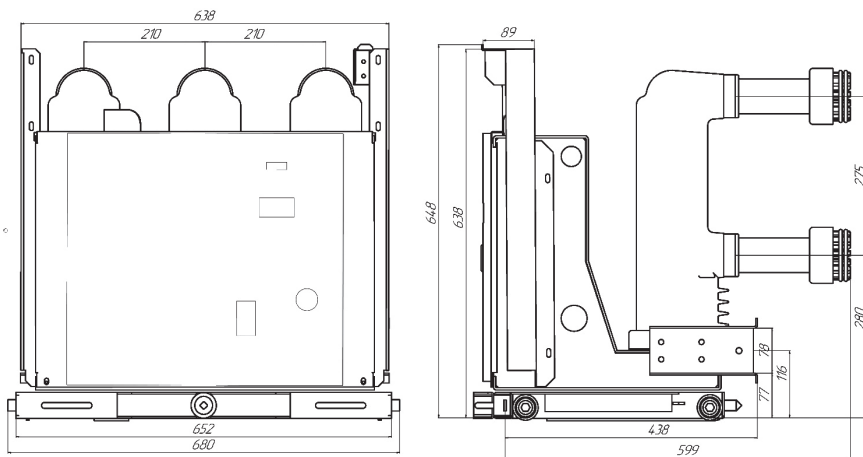
Рисунок В.2 – Габаритные, присоединительные и установочные размеры выключателя типа (передняя панель не изображена) OptiMat ВВ-MD-10-20 (25; 31,5; 40; 50)/630 (1000; 1250; 1600)-2-МВ (ММ)-210
