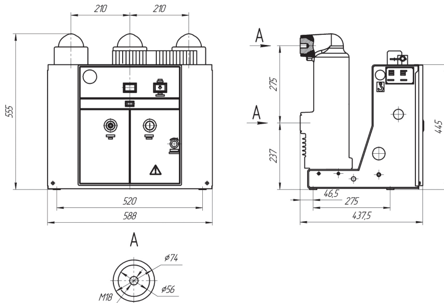
Рисунок А.2 – Габаритные, присоединительные и установочные размеры, масса выключателя типа OptiMat ВВ-MD-10-20(25; 31,5)/630(1250; 1600)-2-FX -210
