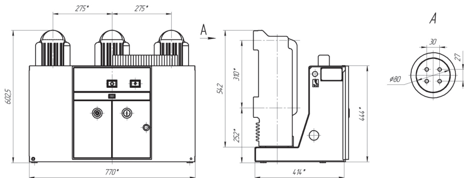
Рисунок А.4 – Габаритные, присоединительные и установочные размеры, масса выключателя типа ВВ-MD-10-31,5 (40; 50)/2000-2-FX-275
