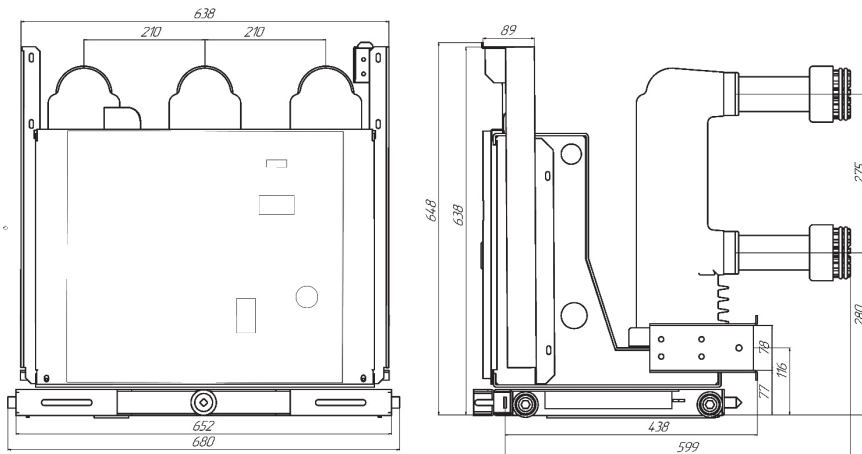
Рисунок В.3 – Габаритные, присоединительные и установочные размеры выключателя типа, передняя панель не изображена OptiMat BB-MD-10-20 (25; 31,5; 40)/2000-2-MB (MM)-210
