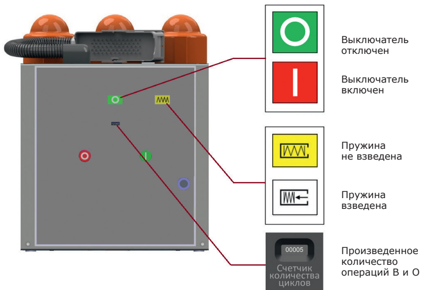
Рисунок 4 – Индикаторы на лицевой панели выключателя
