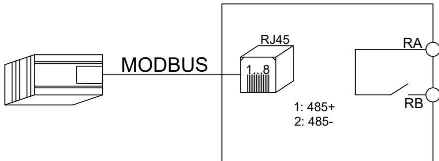
Рисунок 5 — Схема соединений по сети Modbus
