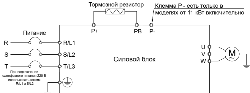
Рисунок 1 – Схема подключения силовых цепей
