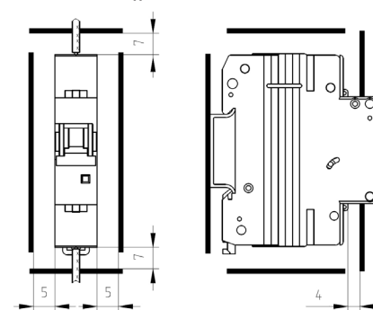
Рисунок И.1 – Минимально допустимые расстояния от выключателя до металлических частей распределительного устройства
