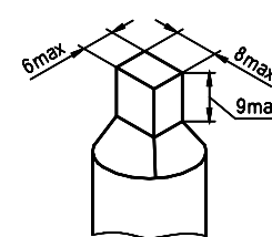
Рисунок Ж.1 – Форма и размеры проводника, подготовленного для присоединения к выключателю
