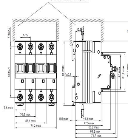
Рисунок В.1 – Габаритные и установочные размеры выключателей на переменный ток
