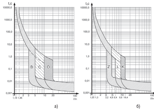
а) характеристики B, C, D; б) характеристики Z, L, K
