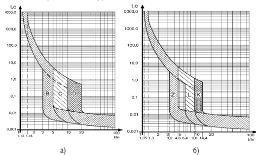
а) характеристики B, C, D; б) характеристики Z, L, K
