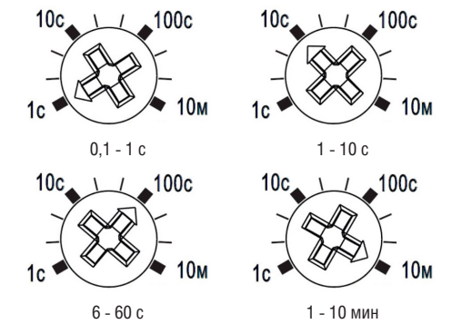
Рисунок 3.3 — Диапазоны выдержки реле
