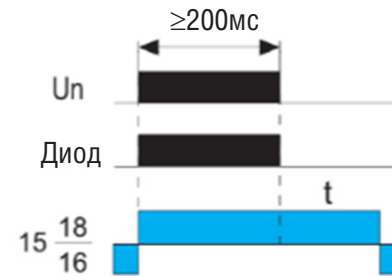
Рисунок 3.2 — Функциональные диаграммы работы реле и их описания приведены далее
