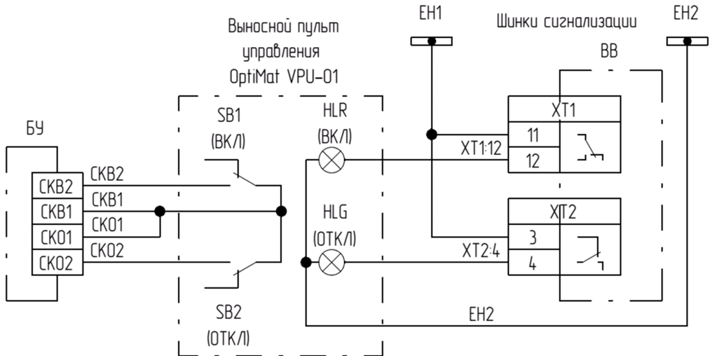
Рисунок 1 – Схема подключения ВПУ
