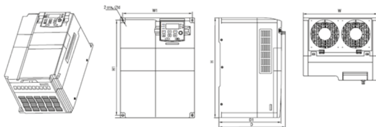
В-15К-Н11К-380-Д-Т, В-18К5-Н15К-380-Д-Т
