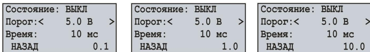
Рисунок 6.25 – Экран настройки значения порога
