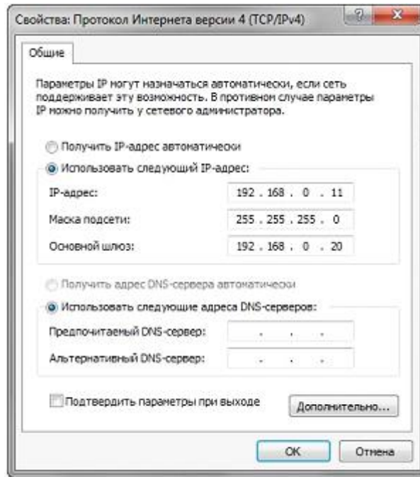
Рисунок А.2 – Пример окна свойств протокола TCP/IPv4 в ОС Windows 7
