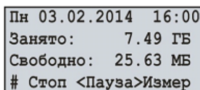
Главный экран (вариант 1)
