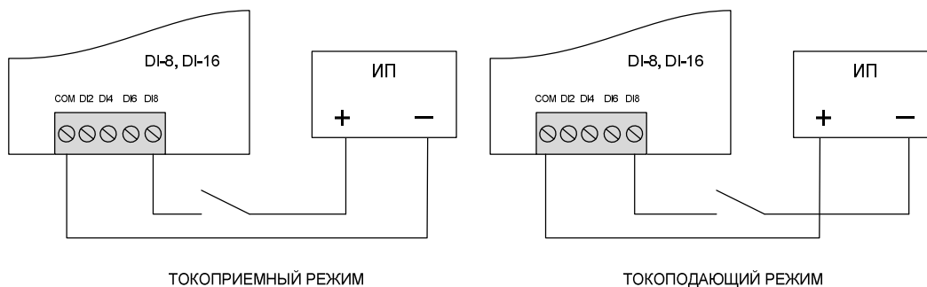
Рисунок 2 - Схема включения цифровых входов в различных режимах
