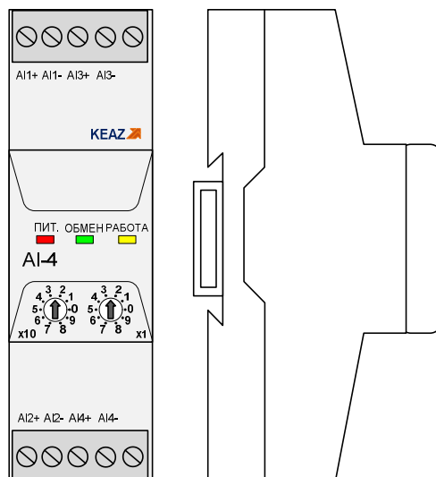
Рисунок 1 – Внешний вид и размеры модуля
