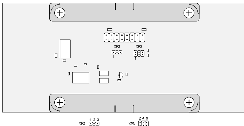
Рисунок 2 – Расположение перемычек XP2 и XP3
