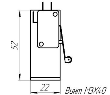
Контакты МП-3
