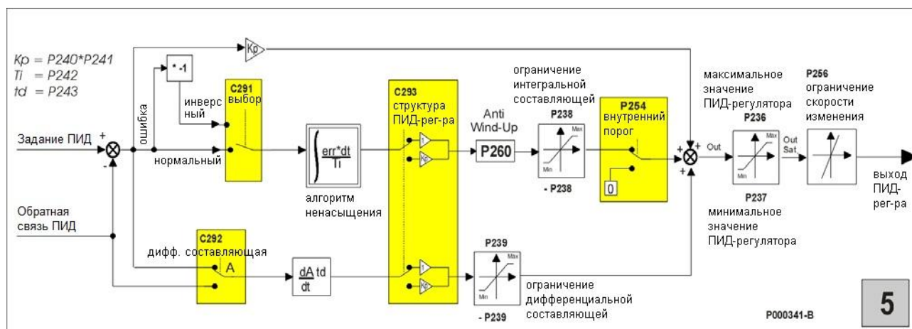
Рис. 23: Блок-схема ПИД-регулятора
