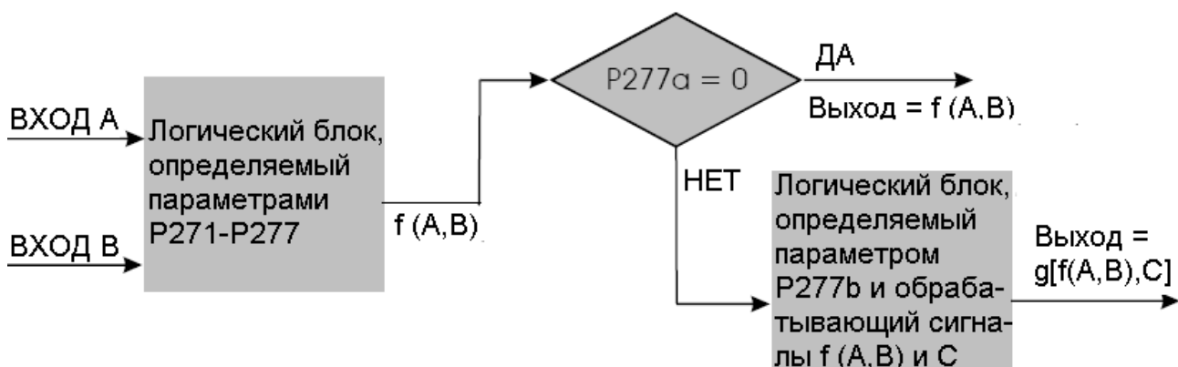
Рис. 31: Блок-схема дискретных выходов
