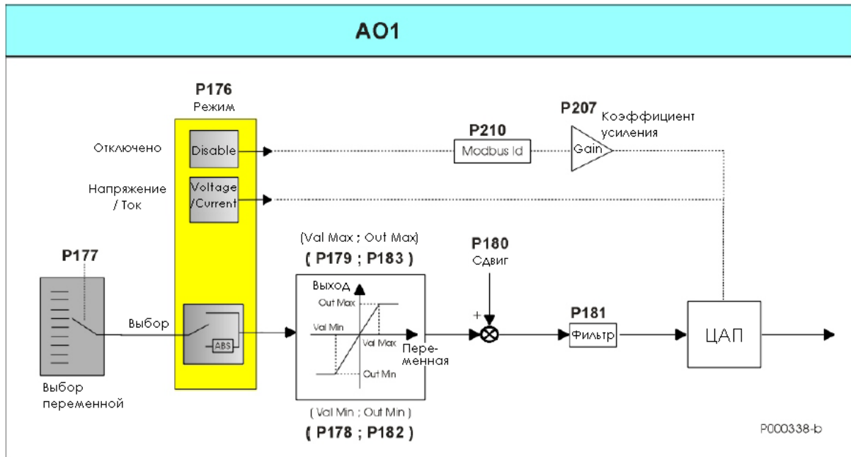
Рис. 15: Общая структура аналоговых выходов
