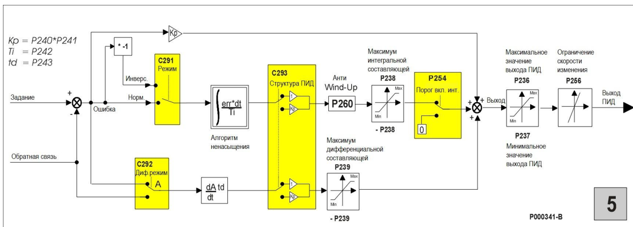
Рис. 66: Структура ПИД-регулятора
