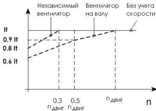
Рис. 60: Снижение тока отключения в зависимости от скорости.
