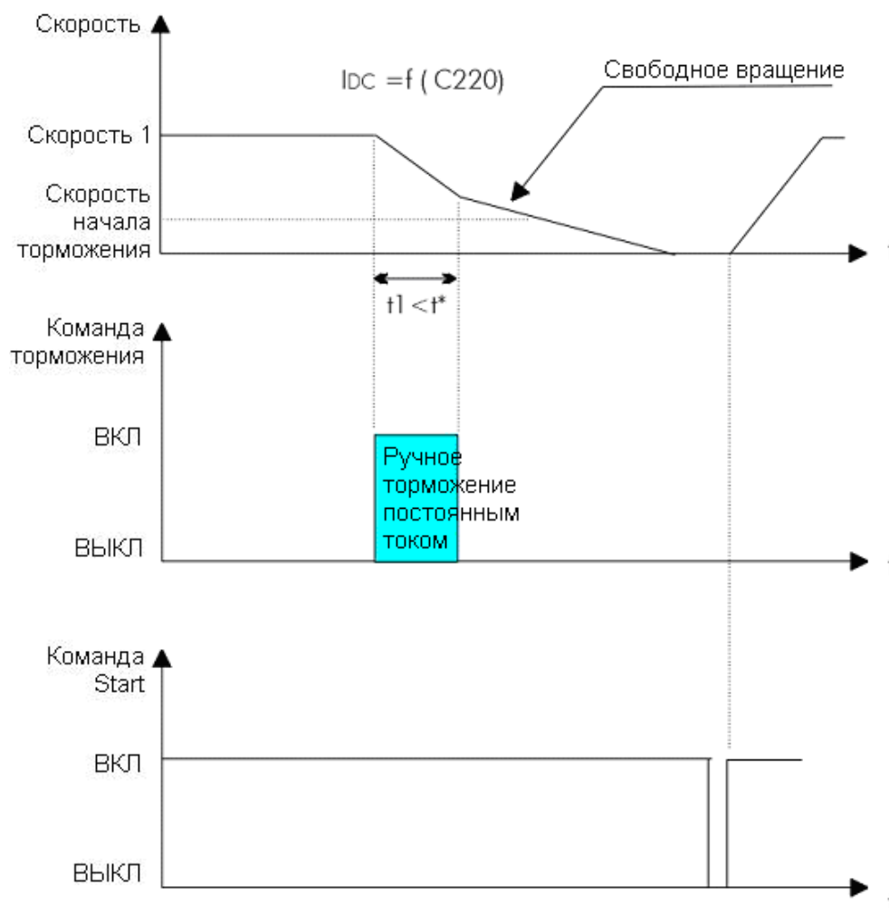
Рис. 55: Ручное торможение (Пример 2). Скорость, торможение, команда торможения и команда START при t1 < t^* и алгоритмах управления IFD или VTC при отключенной функции определения скорости.
