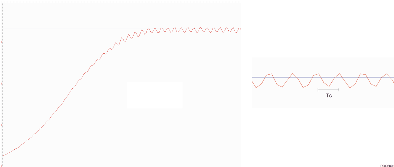
Рис. 24: Постоянные колебания при критическом коэффициенте K_{pc} .
