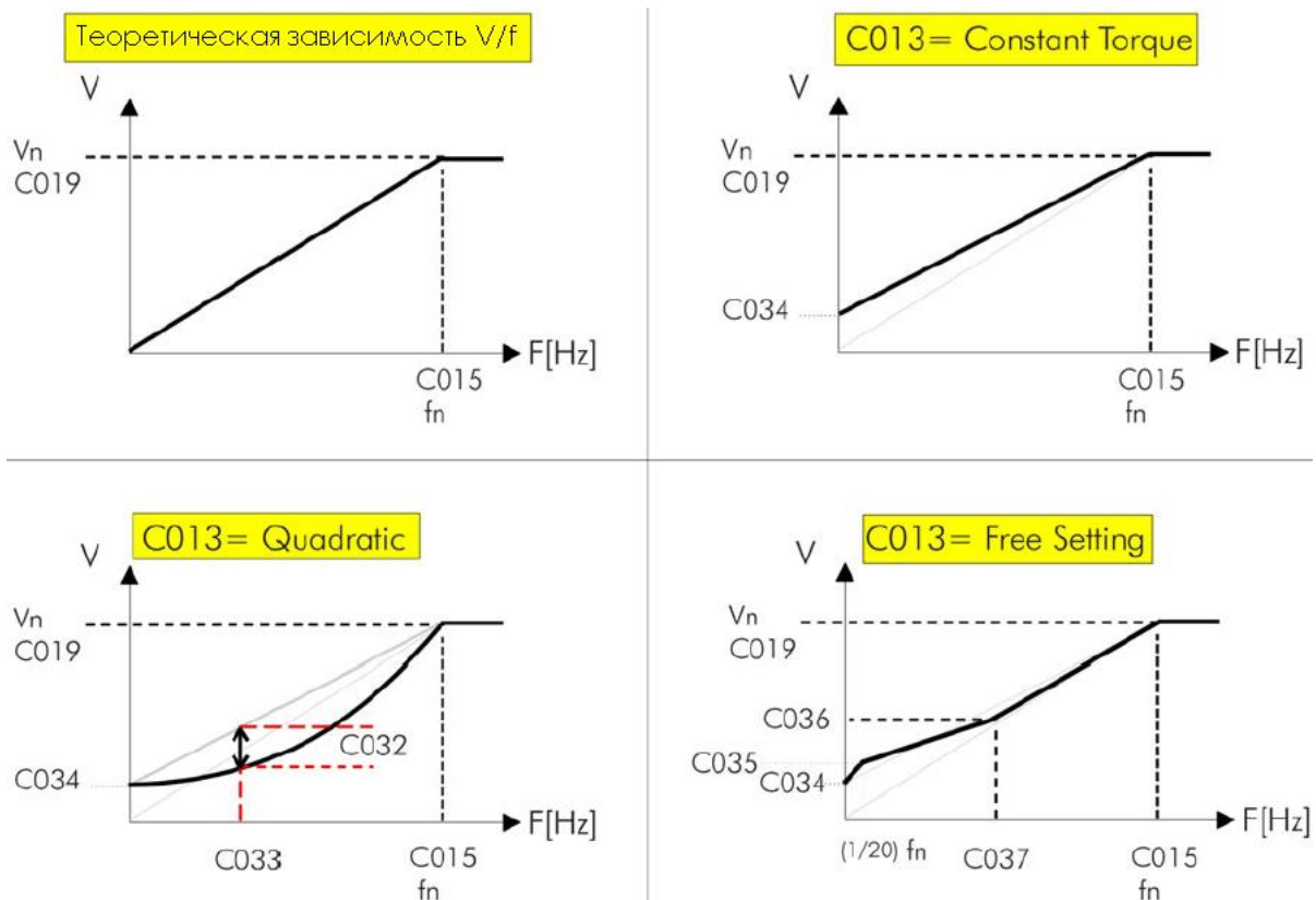
Рис. 42: Типы программируемых зависимостей V/f
