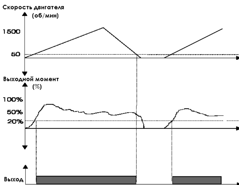
Рис. 37: Управление электромеханическим тормозом (пример)
