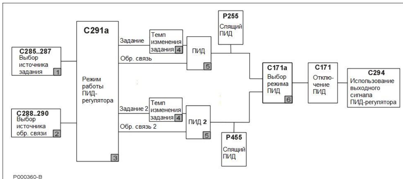
Рис. 63: Структура ПИД-регулятора
