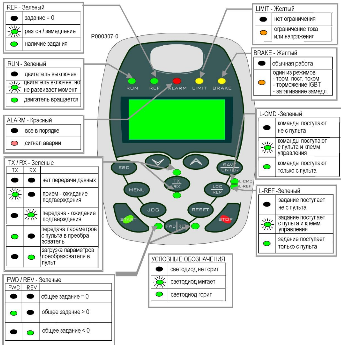
Рис. 3: Пульт управления
