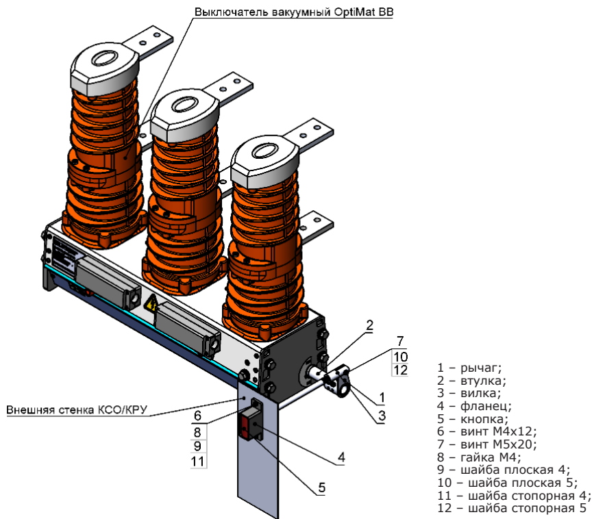
Рисунок А.1 – Пример условного монтажа комплекта КМ-05
