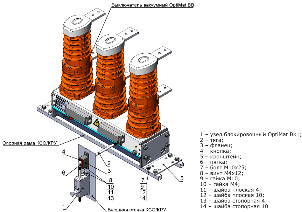
Рисунок А.1 – Пример условного монтажа комплекта КМ-01
