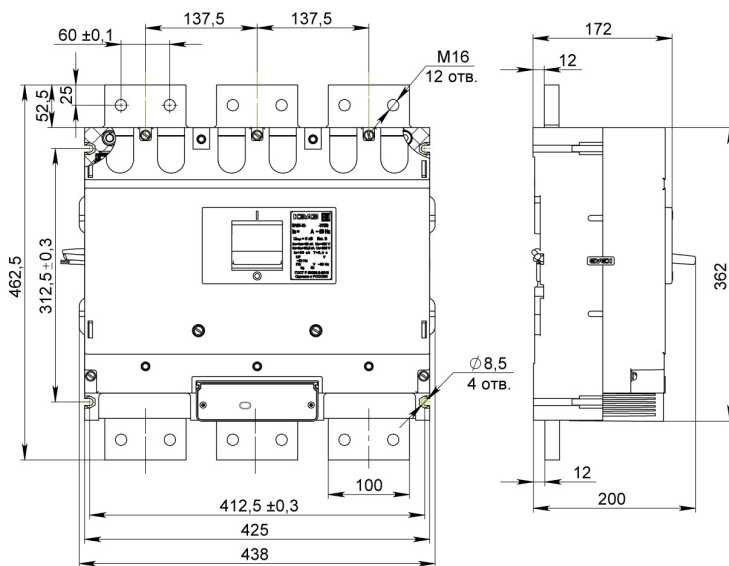
Рисунок Б.1 — Выключатель с ручным приводом на 1600 А
