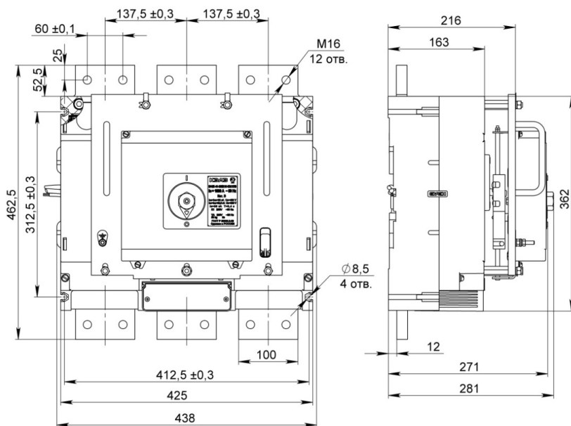
Рисунок Б.2 — Выключатель с электромагнитным приводом на 1600 А
