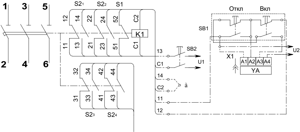
Рисунок Г.3 — Выключатель выдвижного исполнения с дополнительными сборочными единицами
