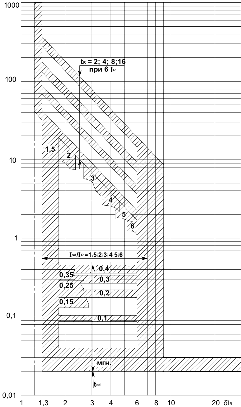
Рисунок В.1 — Выключатель ВА53–43. Обратно-квадратичная зависимость
