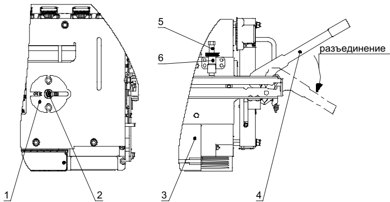
Рисунок 5.7 — Выключатель выдвижного исполнения с ручным дистанционным приводом
