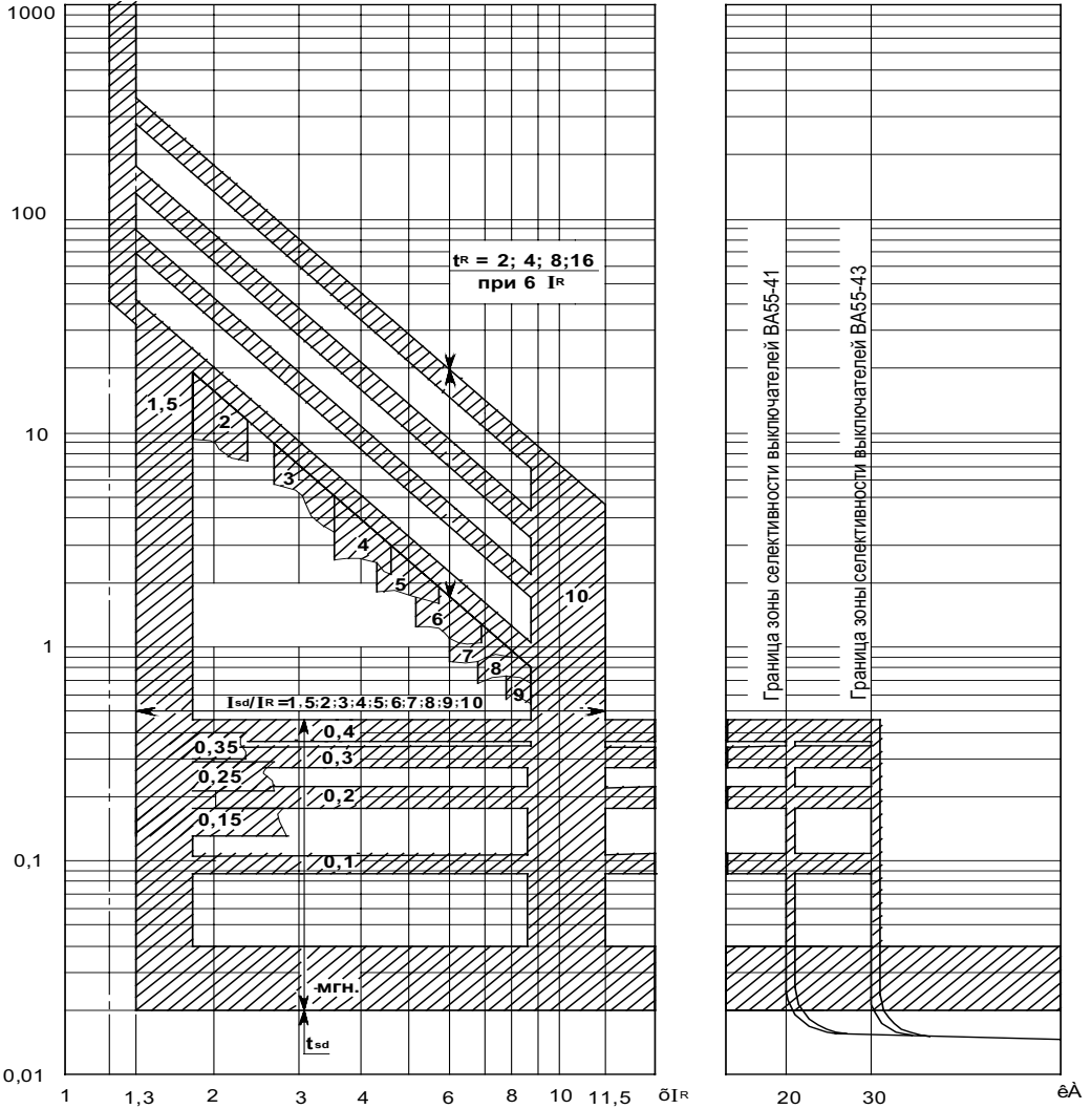
Рисунок В.3 — Выключатель ВА55-43. Обратно-квадратичная зависимость
