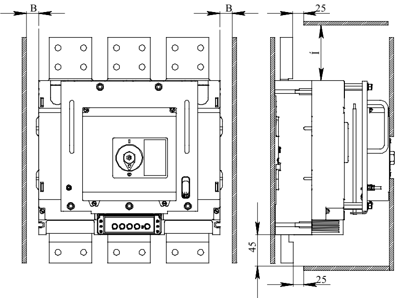
Рисунок Д.2 — Выключатель с электромагнитным приводом
