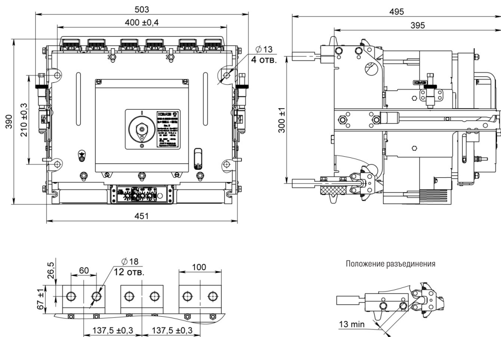
Рисунок 5.5 — Выключатель выдвижного исполнения с электромагнитным приводом
