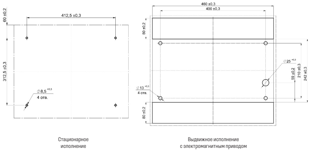
Рисунок 5.8 — Выполнение отверстий в панели для установки выключателя
