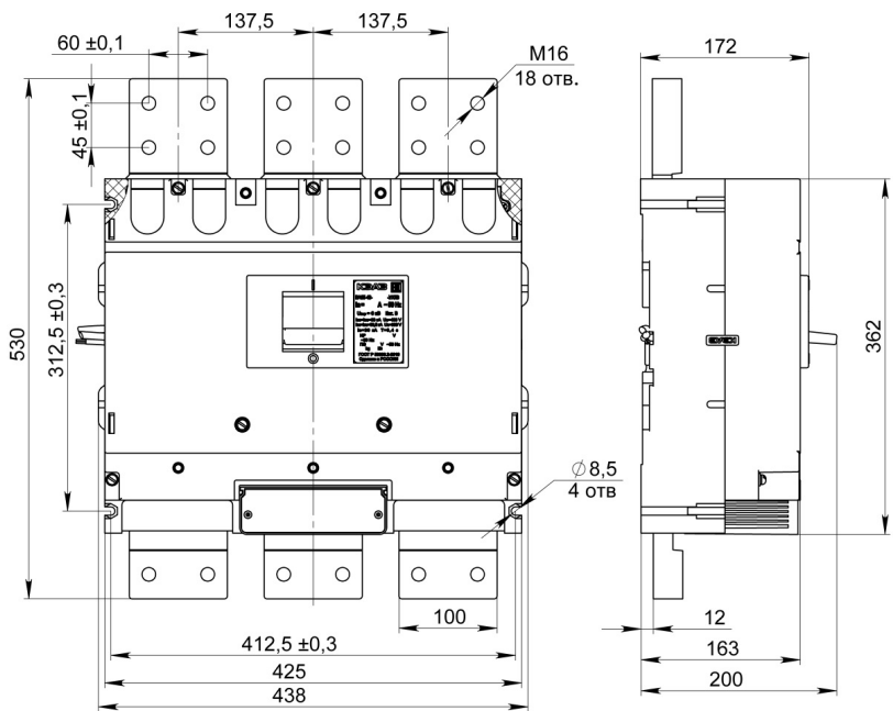
Рисунок Б.3 — Выключатель с ручным приводом на 2000 А
