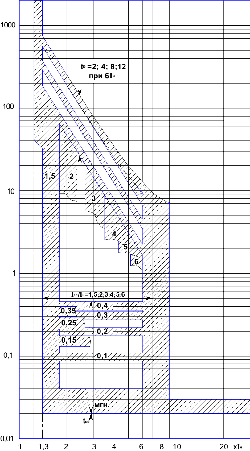
Рисунок В.2 — Выключатель ВА53–43. Обратнo-кубическая зависимость
