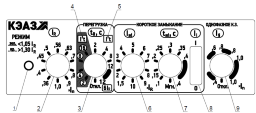
Рисунок 2 — Общий вид лицевой панели ПБМРТ
