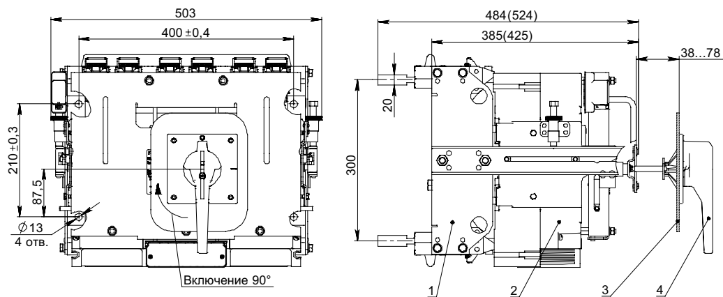
Рисунок 5.6 — Выключатель выдвижного исполнения с ручным дистанционным приводом
