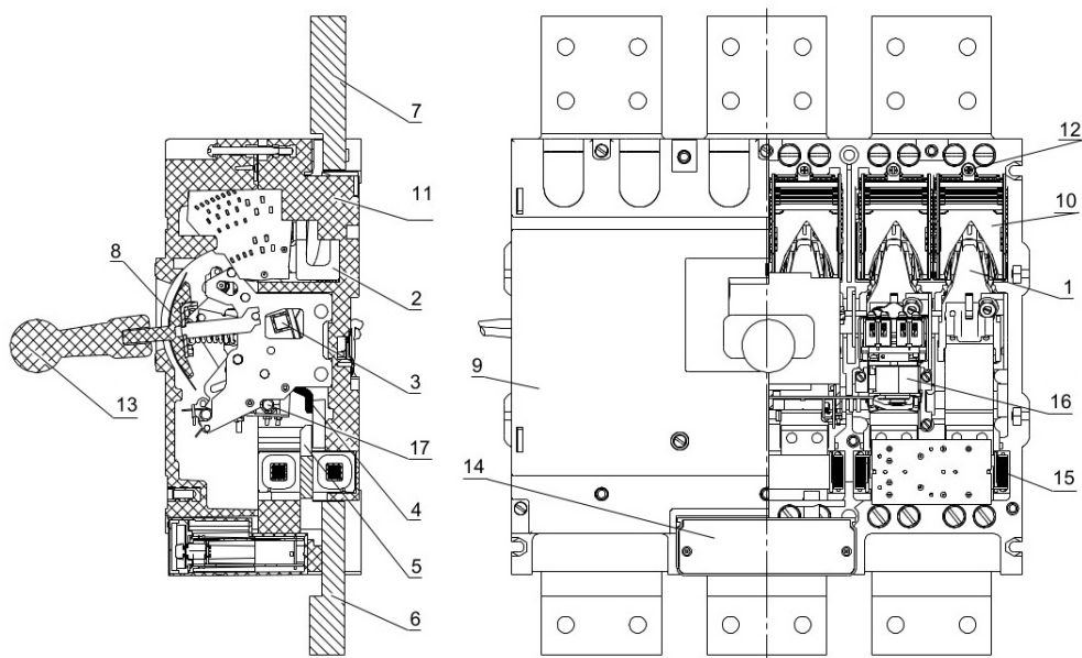
Рисунок 2 — Общий вид лицевой панели ПБМРТ
