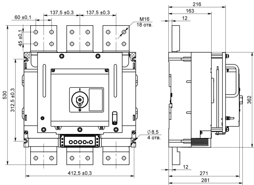
Рисунок Б.4 — Выключатель с электромагнитным приводом на 2000 А
