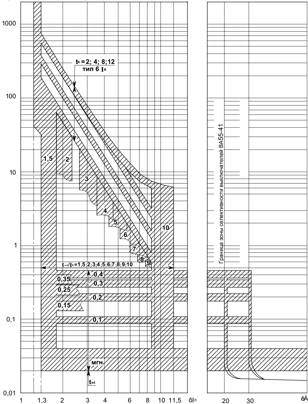
Рисунок В.4 — Выключатель ВА55-43. Обратно-кубическая зависимость
