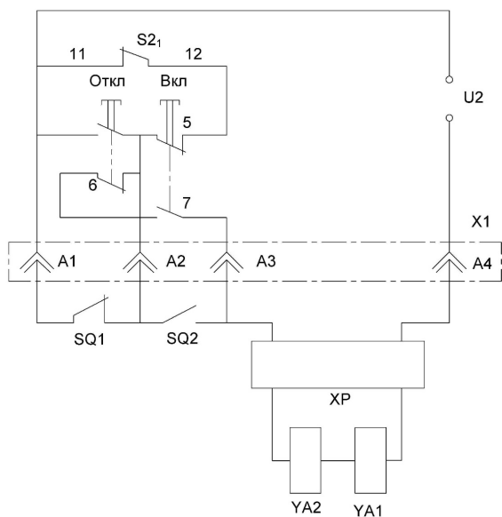
Рисунок Г.5 — Электромагнитный привод постоянного тока
