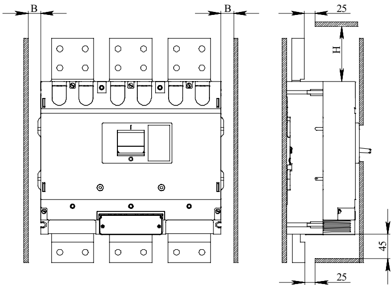
Рисунок Д.2 — Выключатель с электромагнитным приводом
