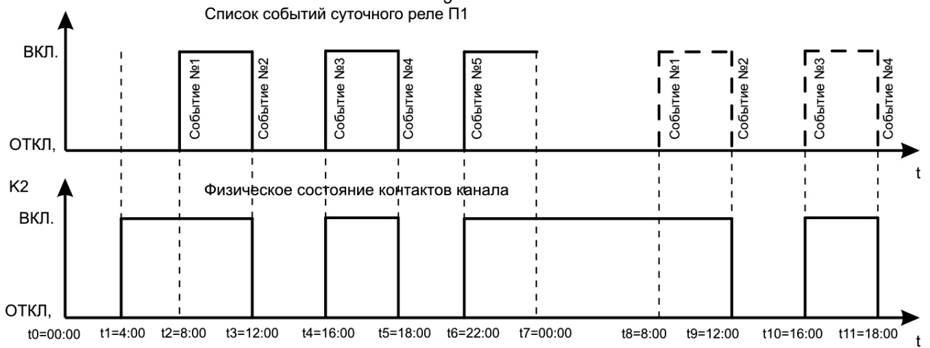
Рисунок 2.8 - Режим циклического выполнения списка таймеров на примере суточного реле времени
