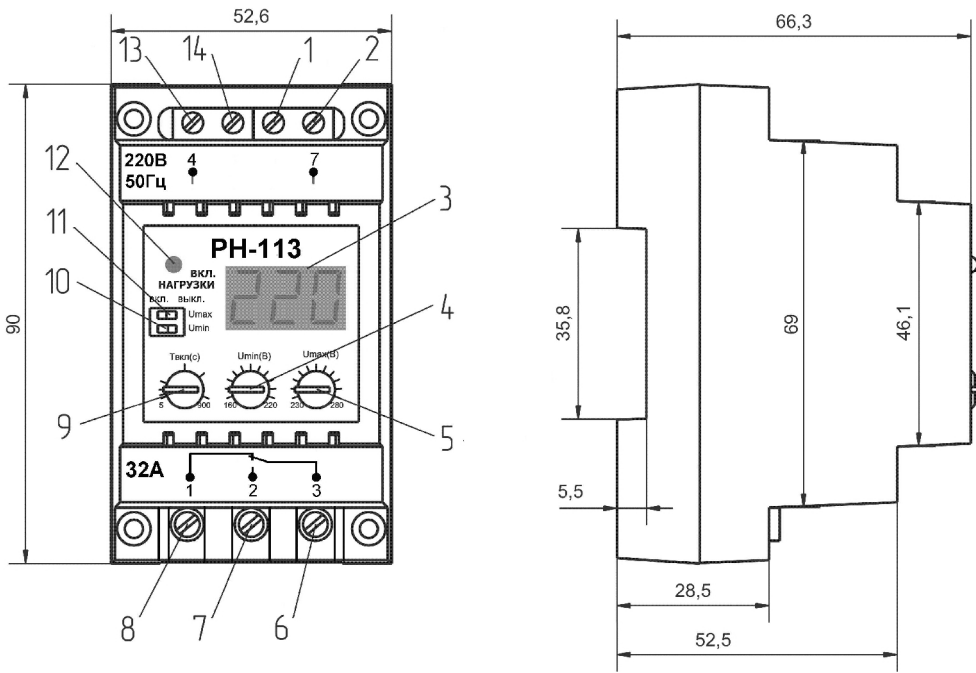
Рисунок 1 – Органы управления, габаритные и установочные размеры OptiDin PH-113
