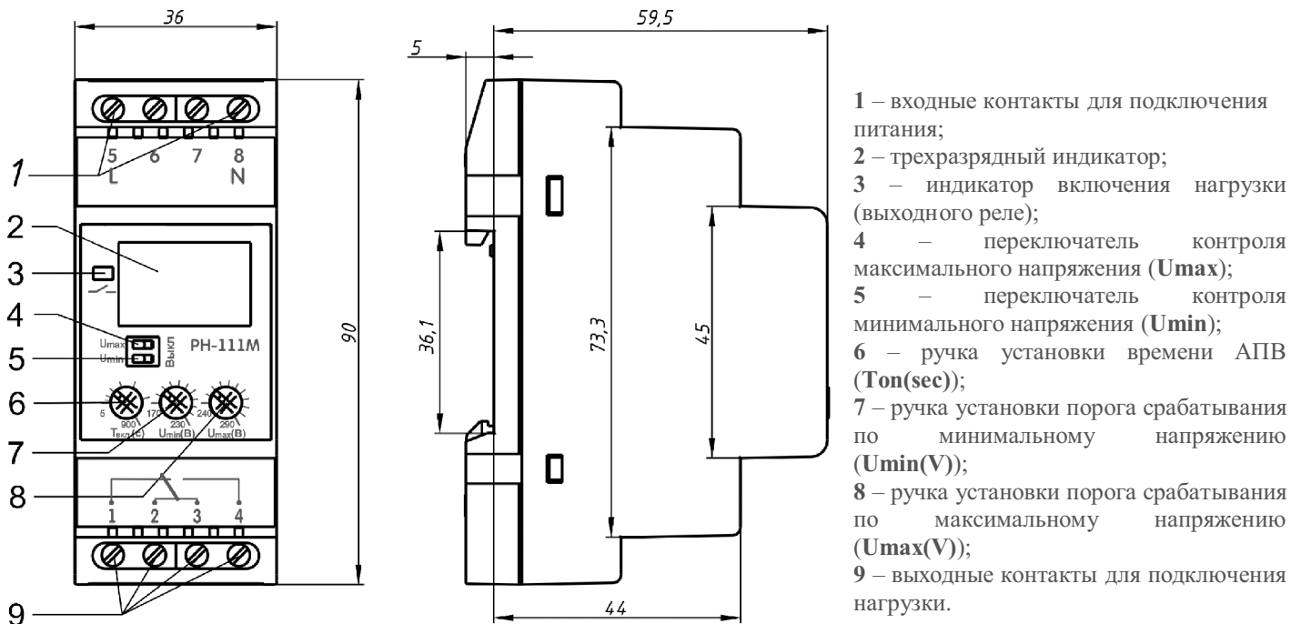
Рисунок 1 – Органы управления, габаритные и установочные размеры OptiDin PH-111M
