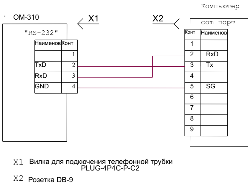
Рисунок 2.2 - Схема подключения OptiDin OM-310 к компьютеру
